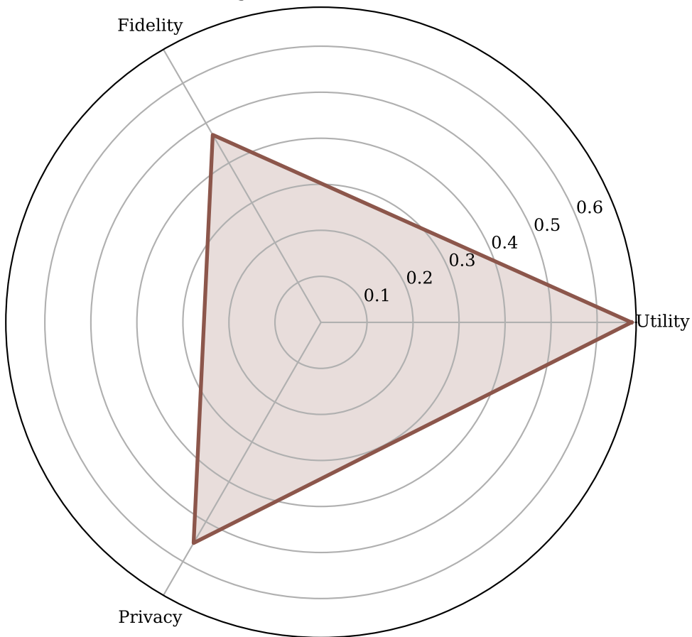
Figure 5: CTABGAN
