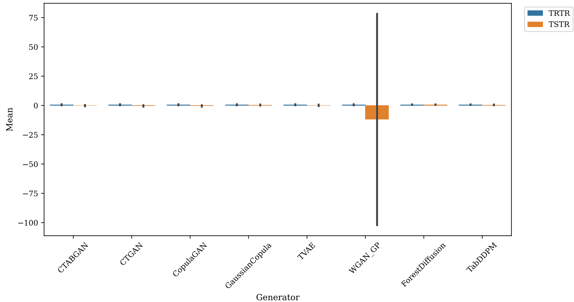
R 2 : TRTR vs TSTR
