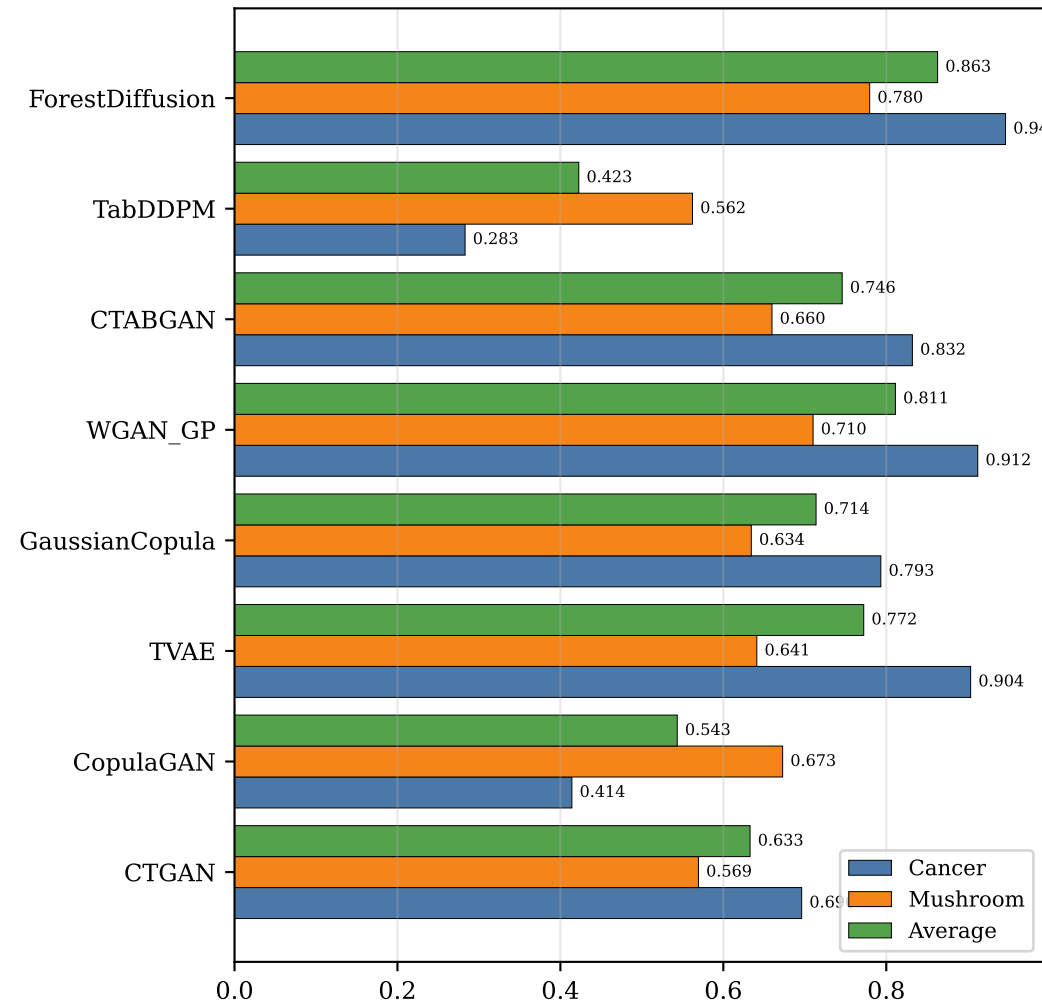
Mean F1
