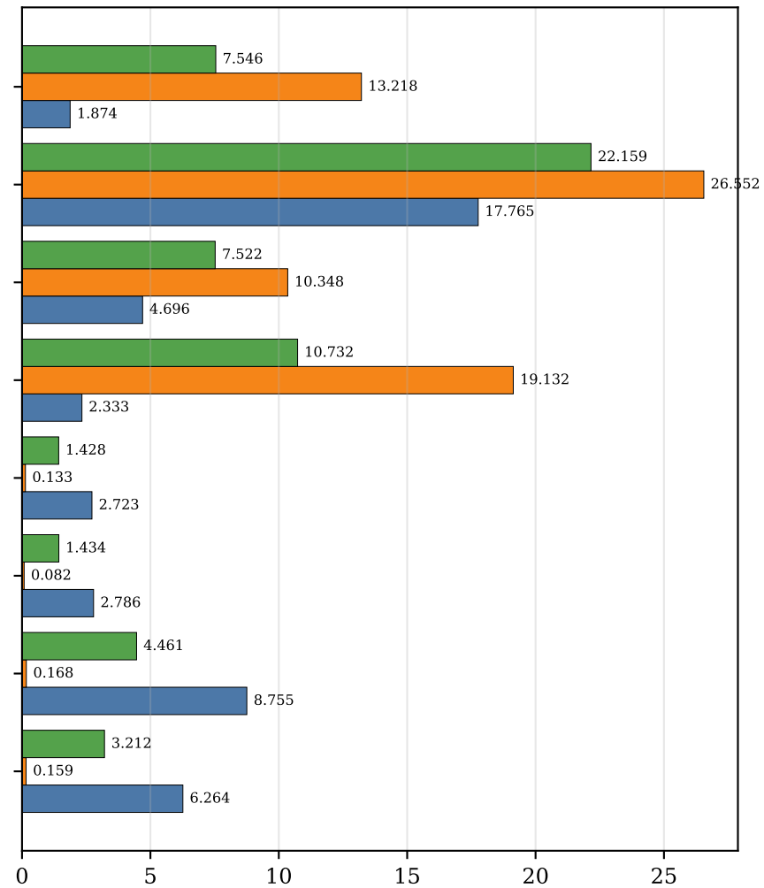
Mean NNDR
