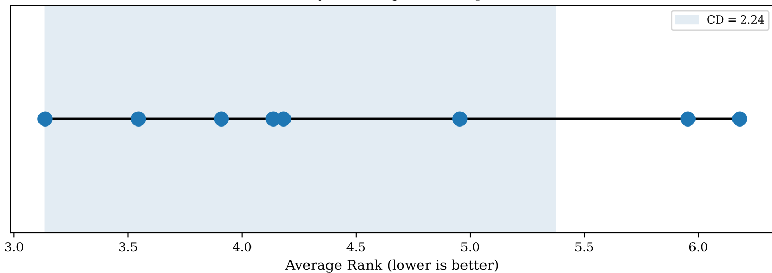
Nemenyi CD Diagram: Composite
