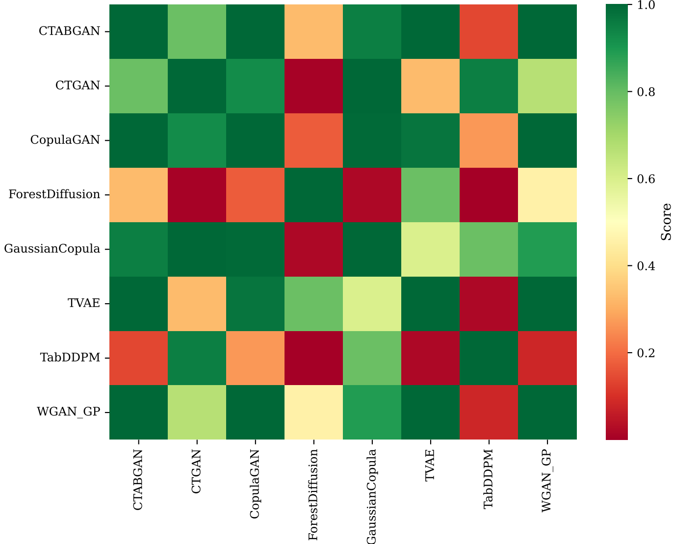
Nemenyi p-matrix: F1
