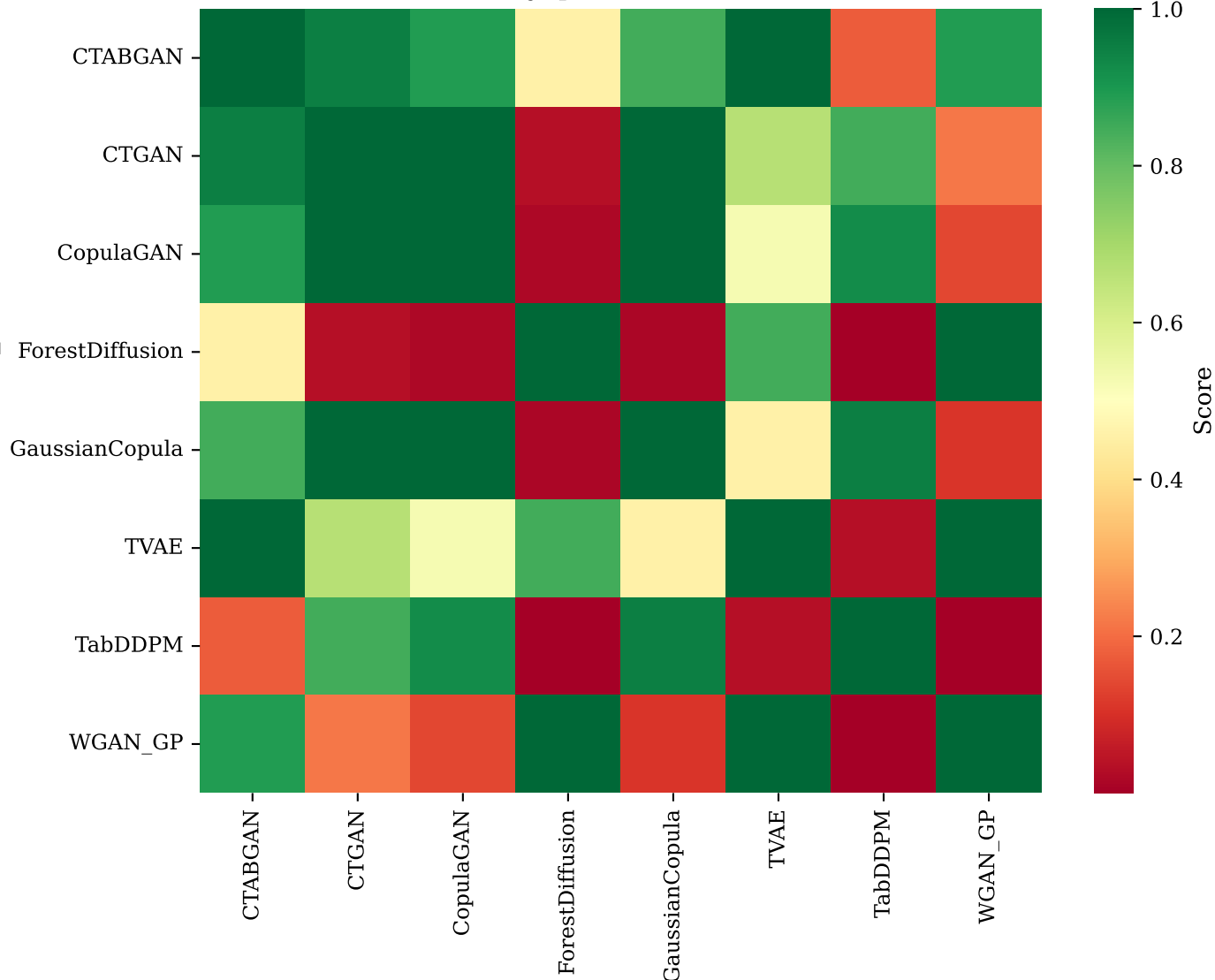
Nemenyi p-matrix: Precision
