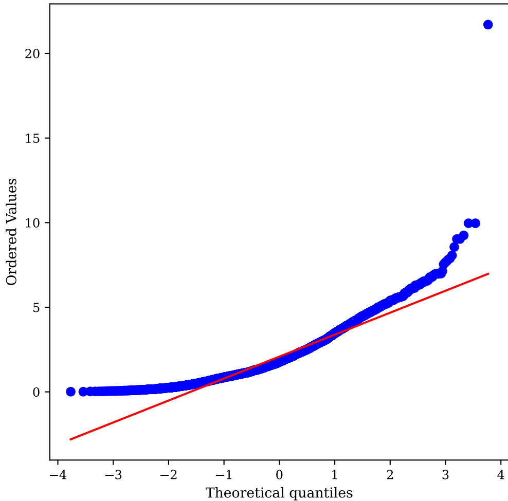
QQ Plot: CTABGAN Mahalanobis
