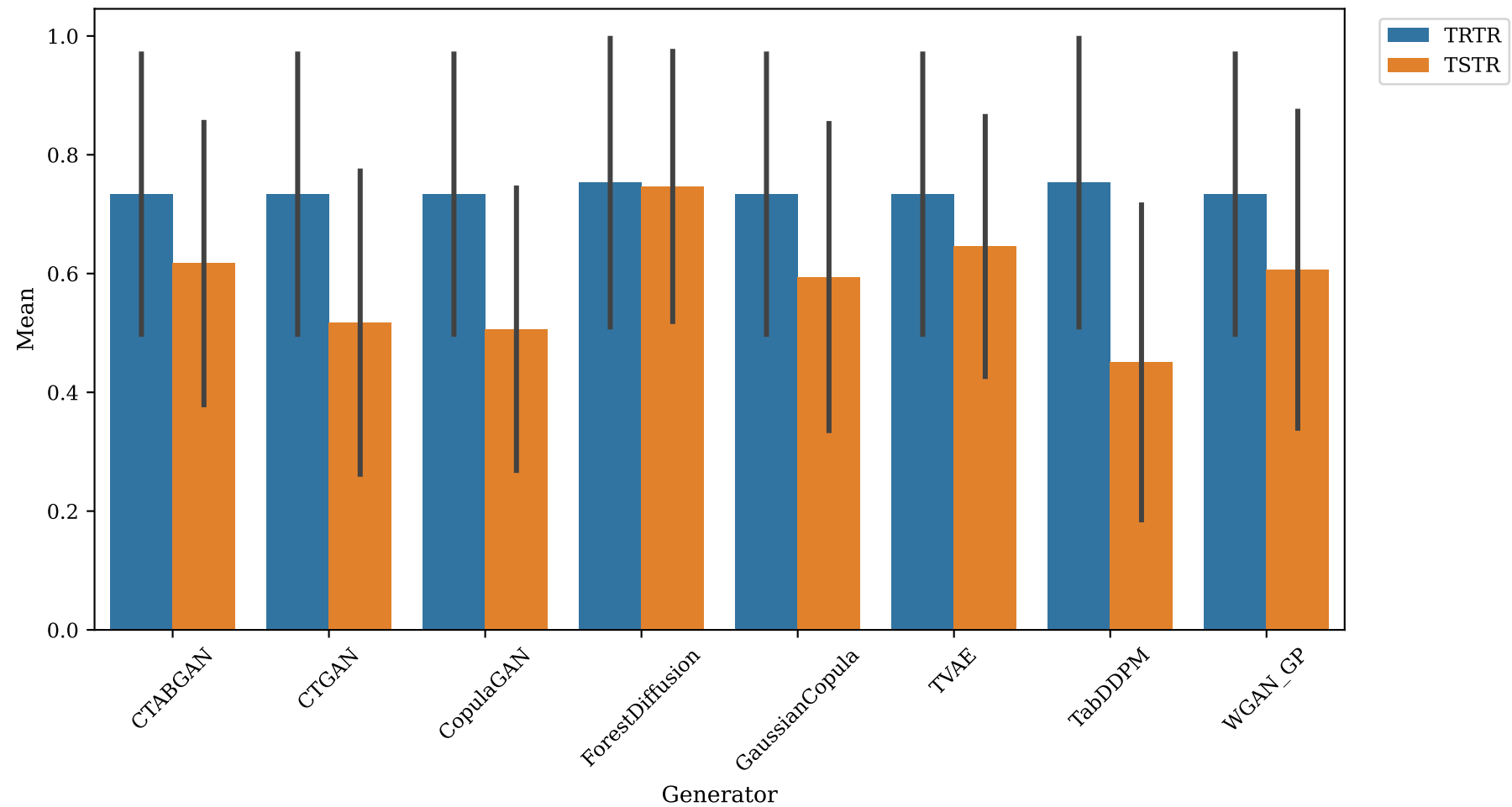
F1: TRTR vs TSTR
