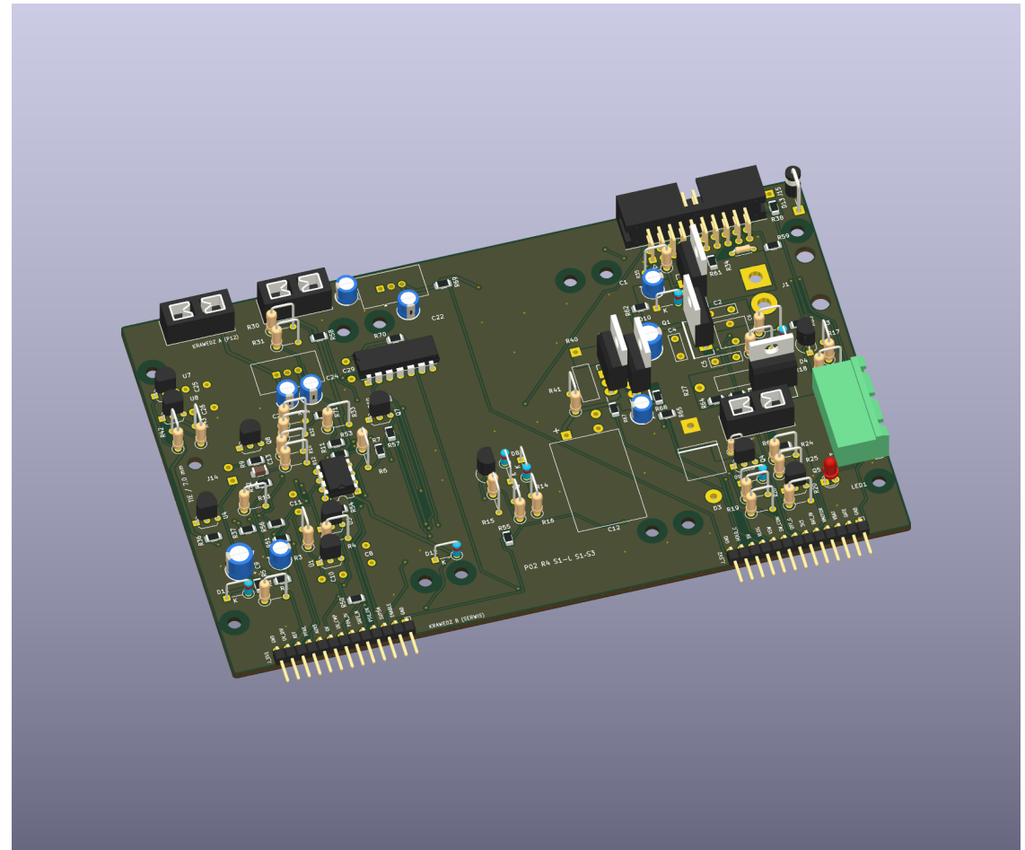
Render KiCad z modelami bibliotecznymi (C_H leżący i pigtaile bez modeli 3D).
