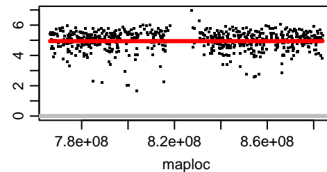
Chromosome OZ183628.2
