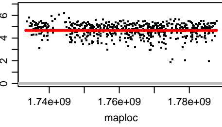
Chromosome OZ183639.2
