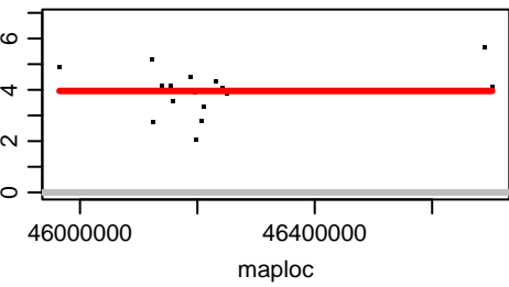
Chromosome OZ183628.2
