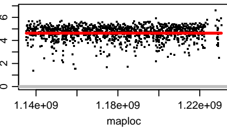
Chromosome OZ183639.2
