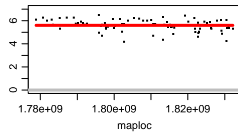
Chromosome OZ183639.2
