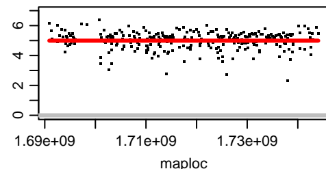
Chromosome OZ183639.2
