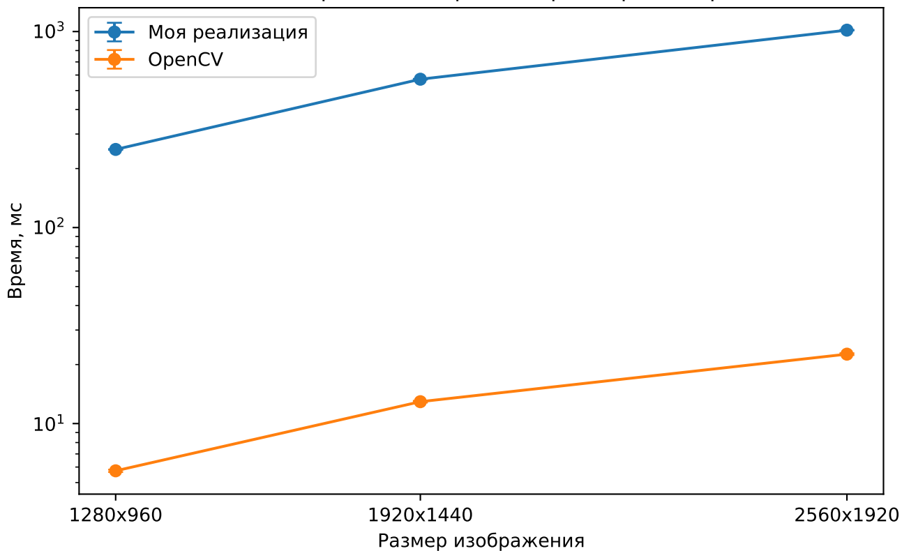
Сравнение времени свёртки
