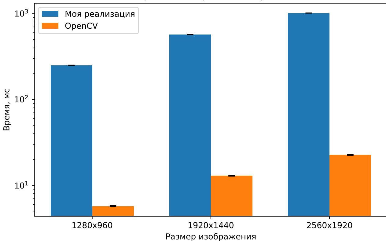
Сравнение времени свёртки
