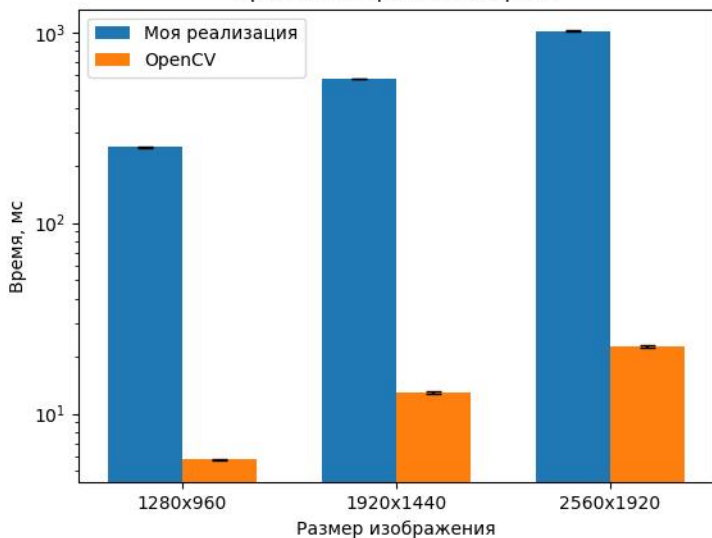
Сравнение времени свёртки
