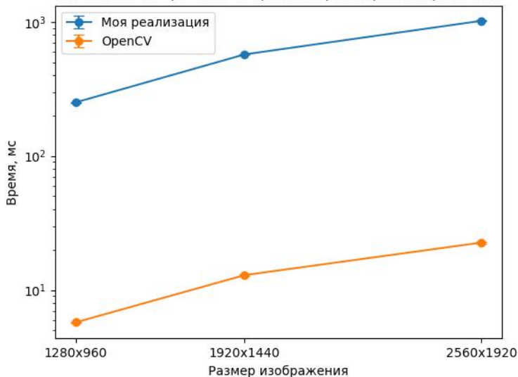
Зависимость времени свёртки от размера изображения
