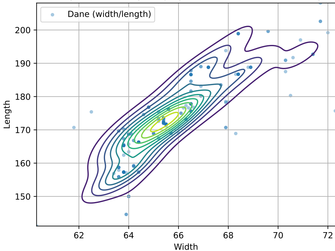
Dwuwymiarowa estymacja gęstości KDE dla width i length
