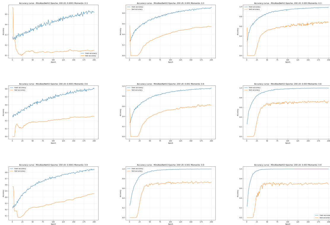
Figura 8: Confronto delle curve di accuratezza per diverse combinazioni di Learning Rate e Momento su MiniAlexNetV2
