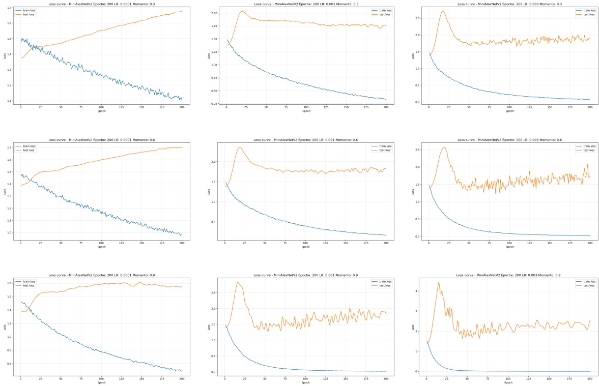
Figura 9: Confronto delle curve di loss per diverse combinazioni di Learning Rate e Momento su MiniAlexNetV2
