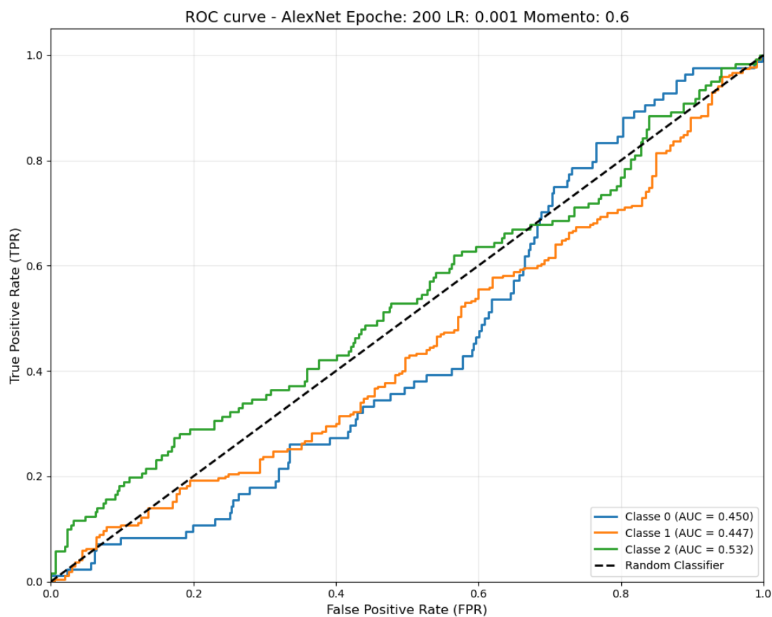
Figura 21: Curve ROC della rete AlexNet.
