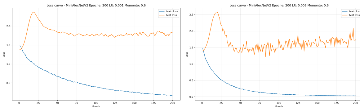
Figura 9: Confronto delle curve di loss per diverse combinazioni di Learning Rate e Momento su MiniAlexNetV2
