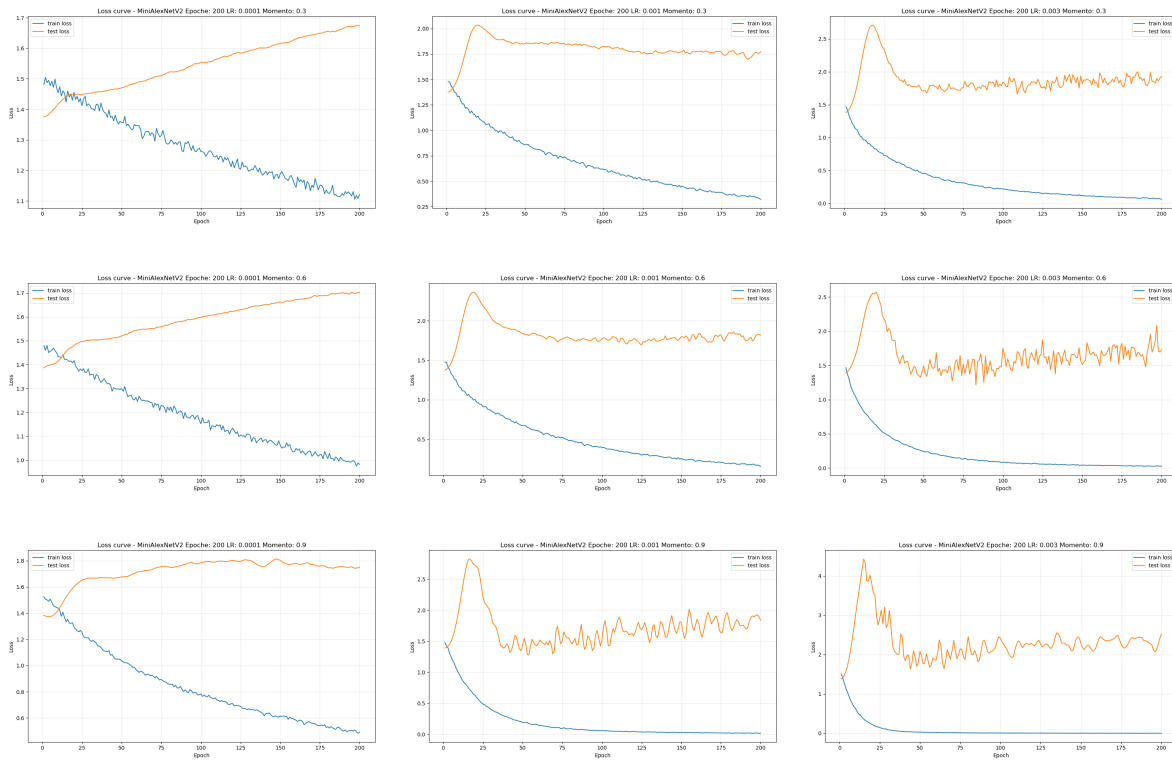
Figura 25: Confronto delle curve di loss per diverse combinazioni di Learning Rate e Momento su MiniAlexNetV2
