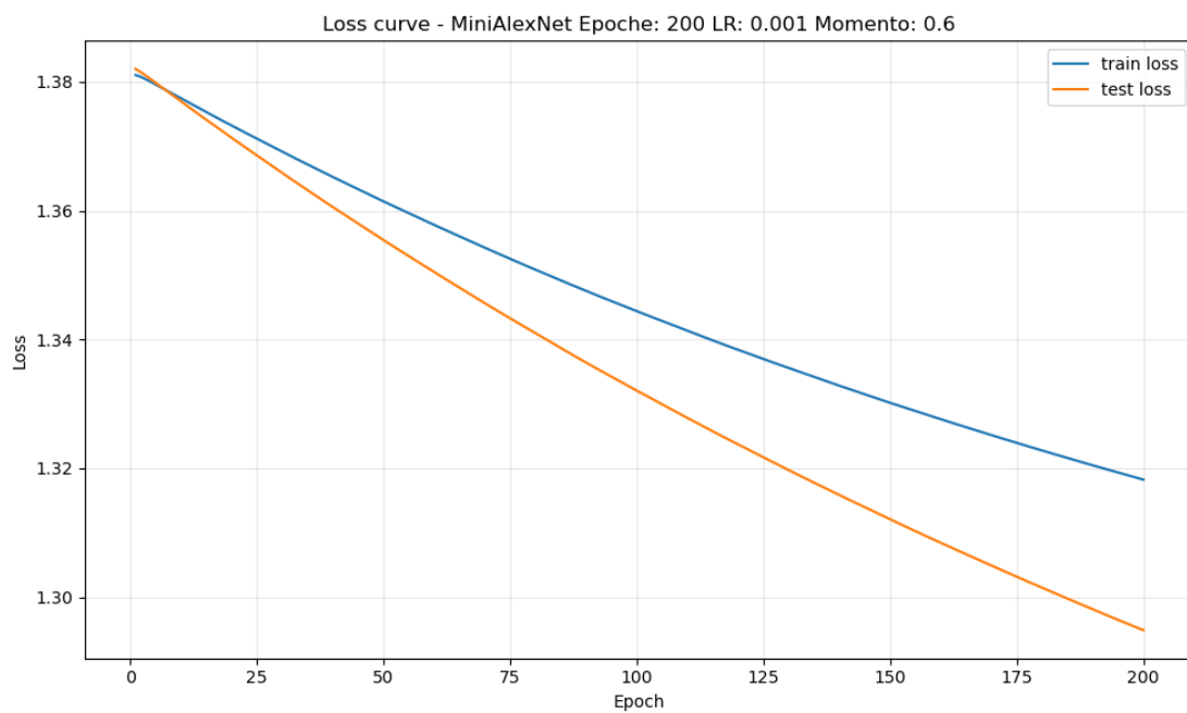
Figura 18: Curva di loss della rete MiniAlexNet.
