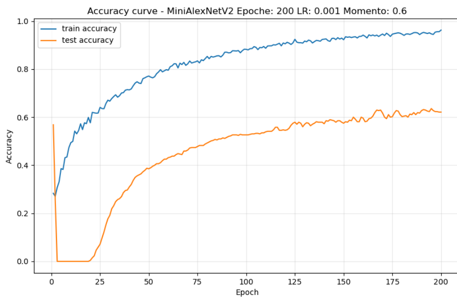
Figura 15: Curva di accuratezza della rete MiniAlexNetV2.
