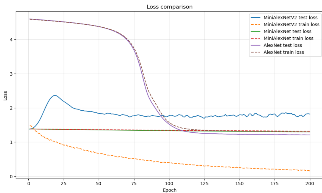
Figura 20: Curve di loss delle reti.
