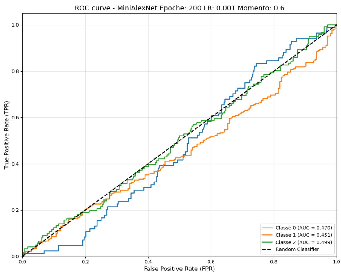
Figura 22: Curve ROC della rete MiniAlexNet.
