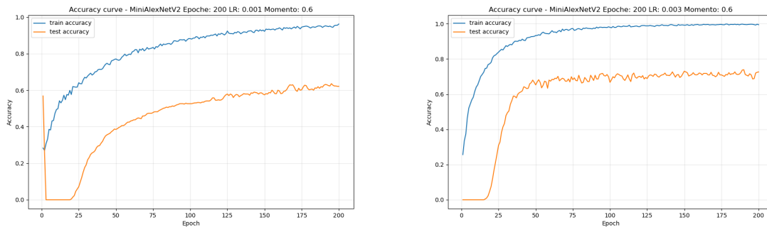
Figura 8: Confronto delle curve di accuratezza per diverse combinazioni di Learning Rate e Momento su MiniAlexNetV2
