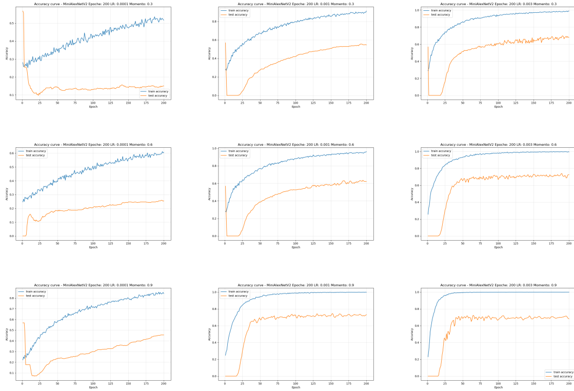
Figura 24: Confronto delle curve di accuratezza per diverse combinazioni di Learning Rate e Momento su MiniAlexNetV2
