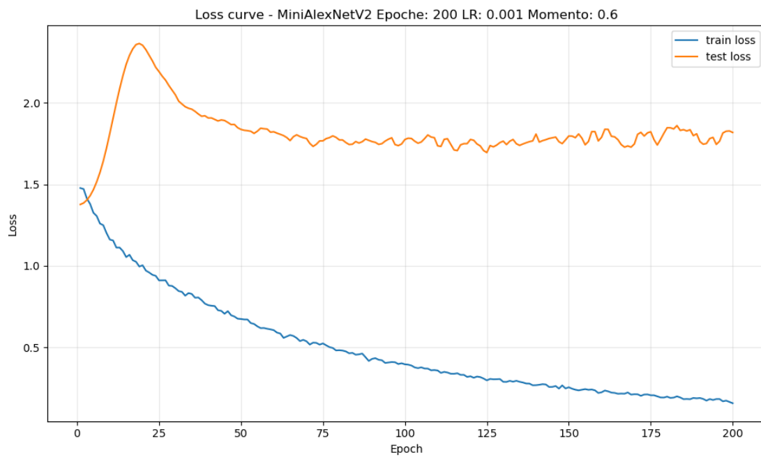
Figura 19: Curva di loss della rete MiniAlexNetV2.
