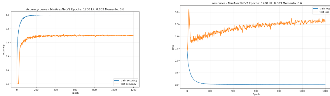
Figura 11: Curve di accuratezza e loss per MiniAlexNetV2 con Learning Rate 0.003, Momento 0.6 su 1200 epoche
