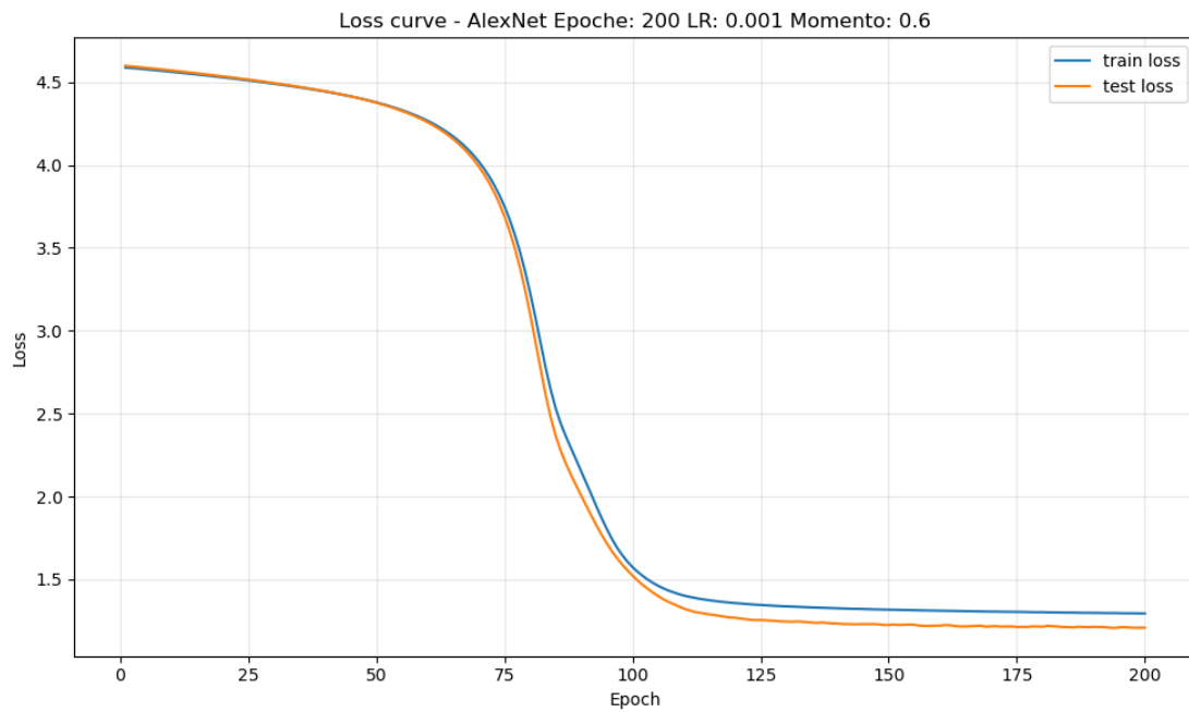
Figura 17: Curva di loss della rete AlexNet.
