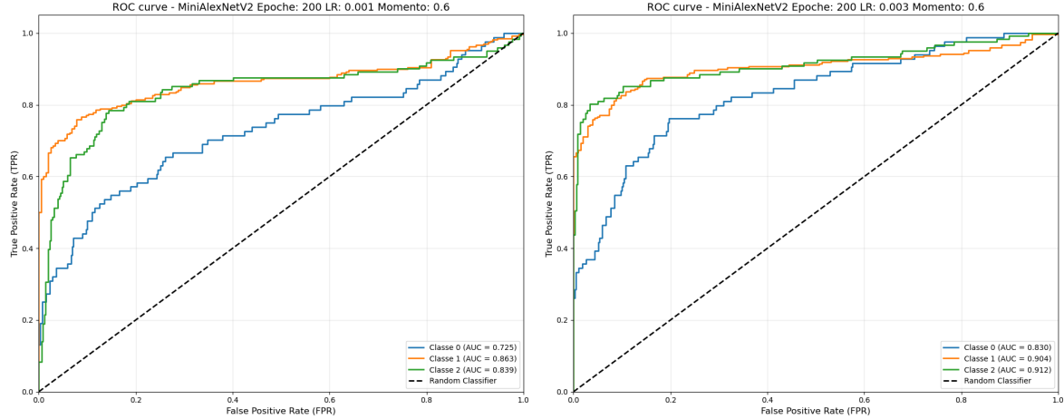
Figura 10: Confronto delle ROC curve per diverse combinazioni di Learning Rate e Momento su MiniAlexNetV2
