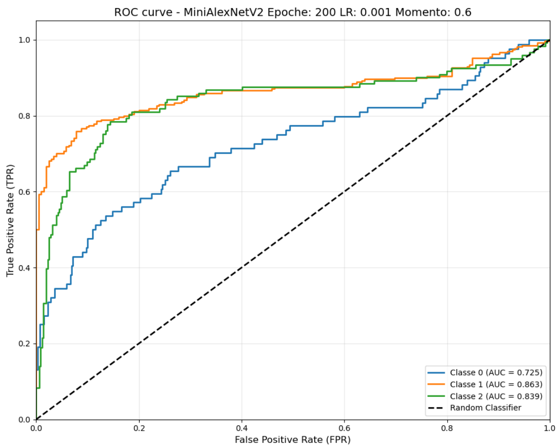
Figura 23: Curve ROC della rete MiniAlexNetV2.
