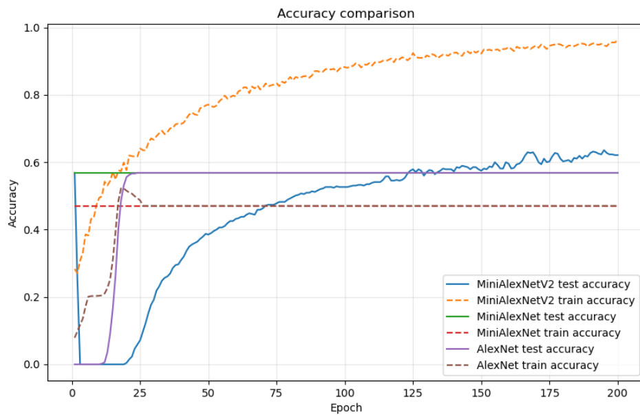
Figura 16: Curve di accuratezza delle reti.
