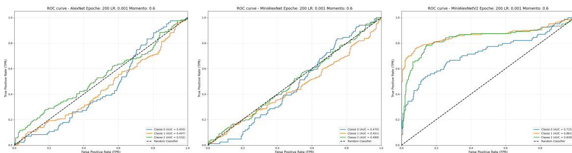
Figura 7: Confronto tra le curve ROC delle tre reti (Learning Rate: 0.001, Momento: 0.6)
