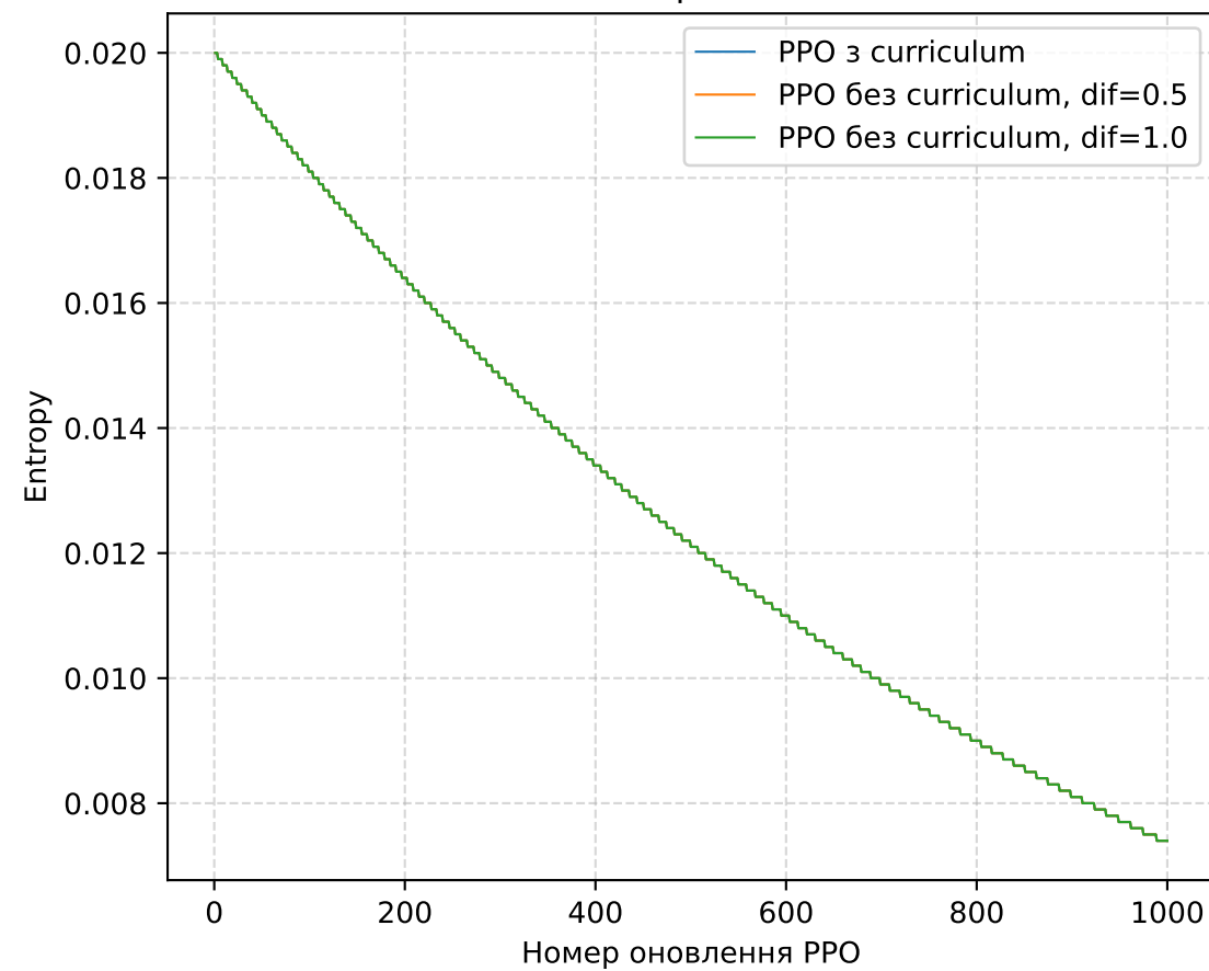
Ентропія
