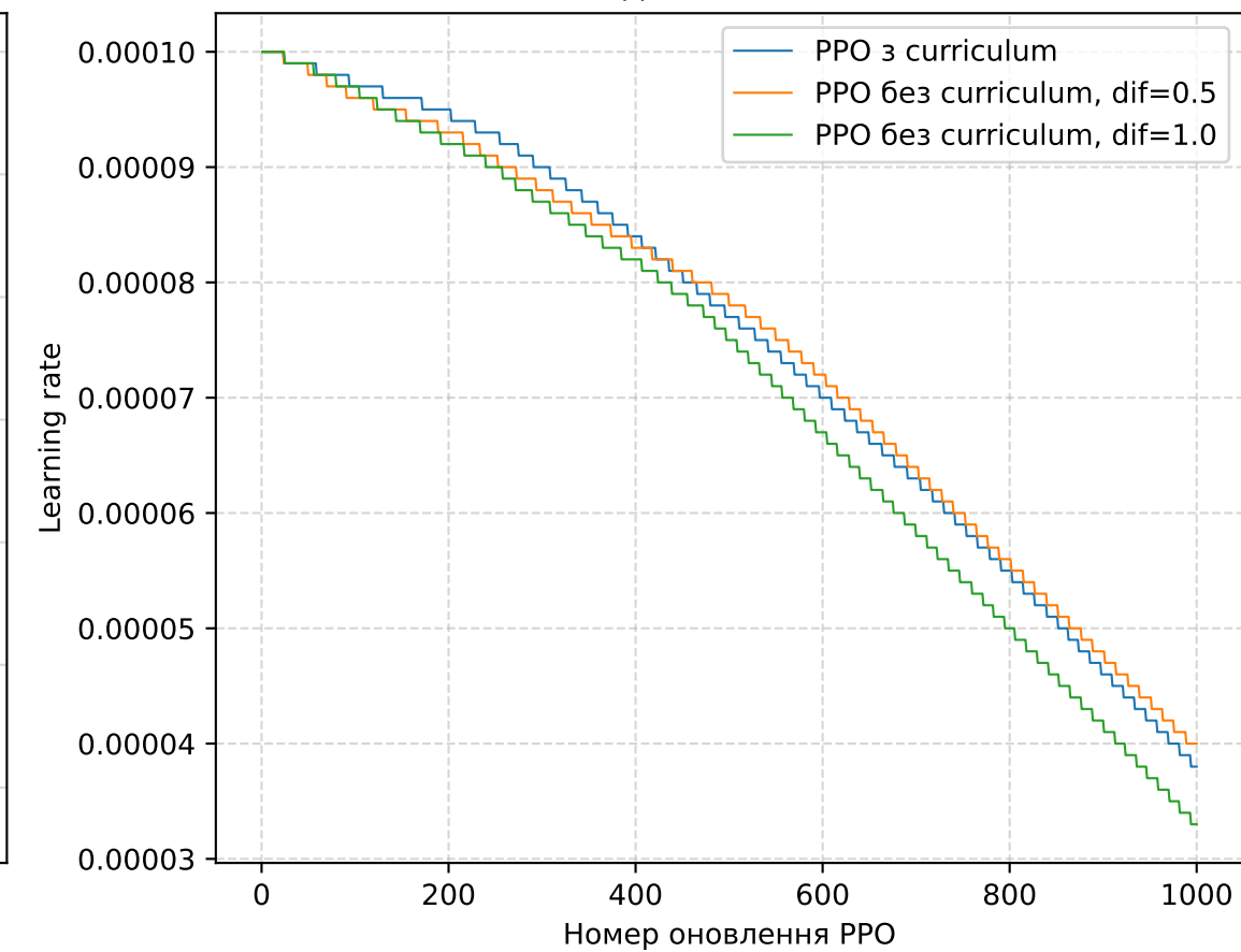
Швидкість навчання
