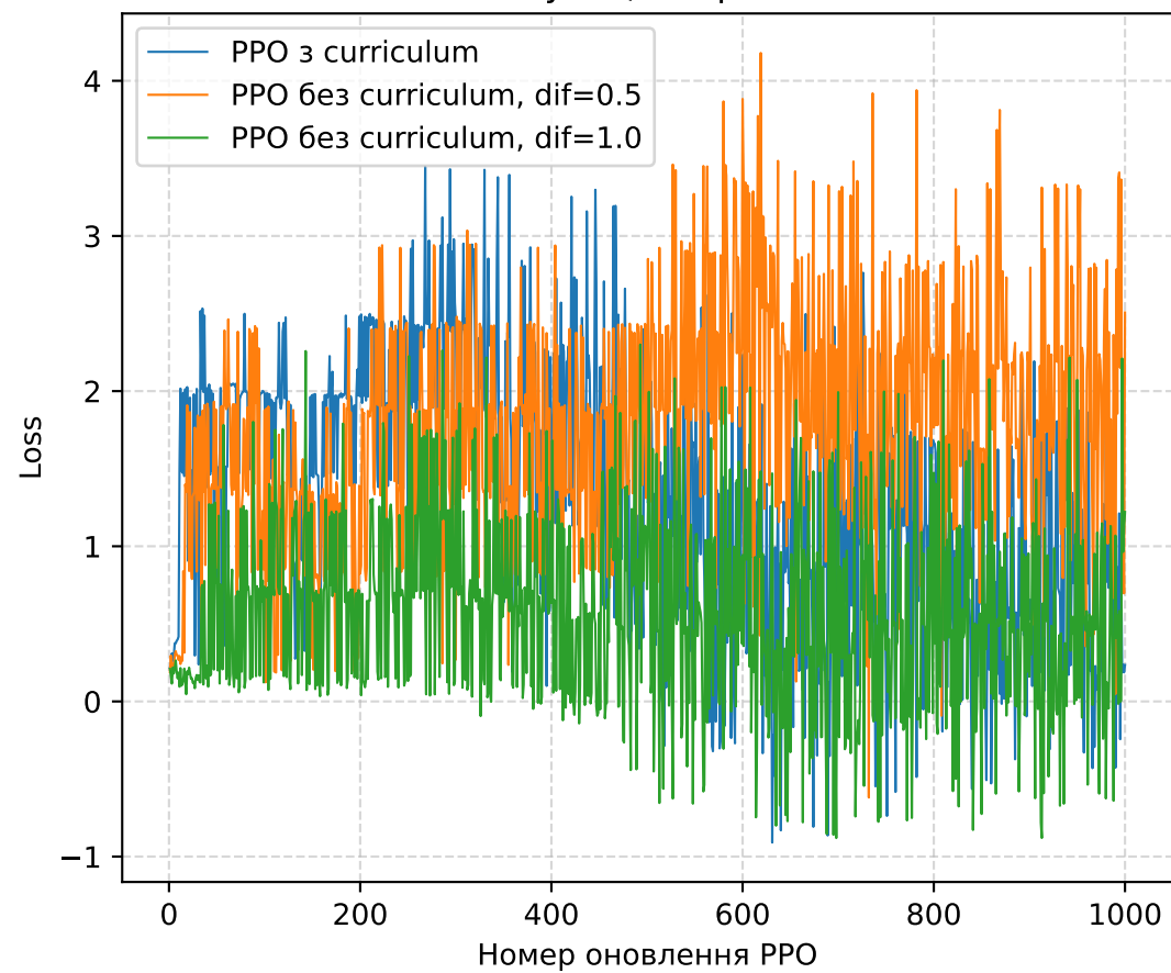
Функція втрат
