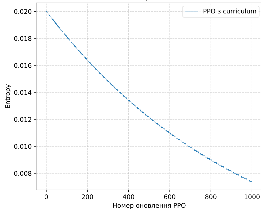
Ентропія
