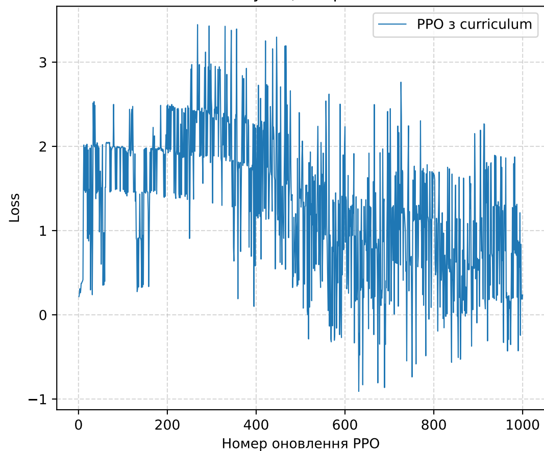
Функція втрат
