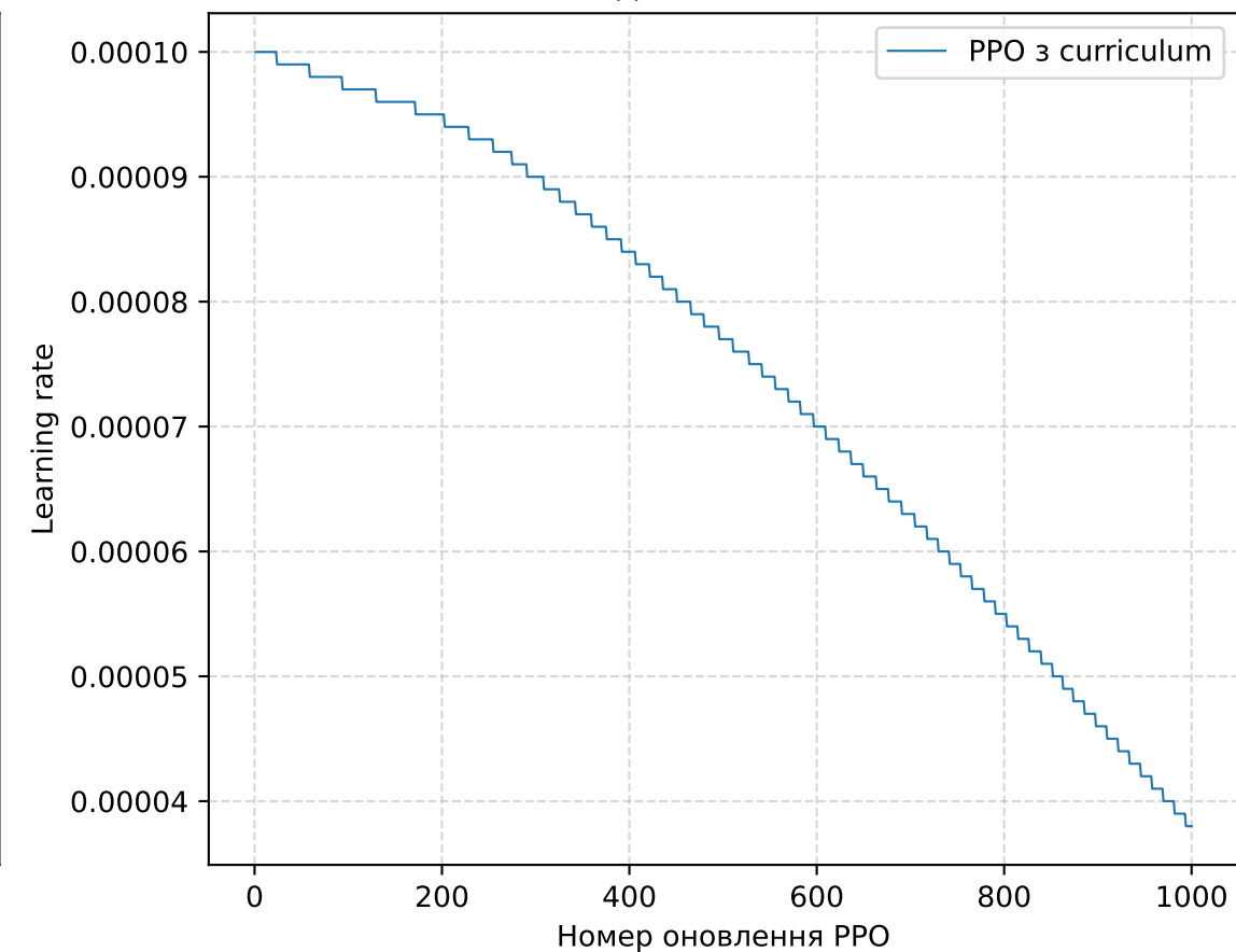
Швидкість навчання
