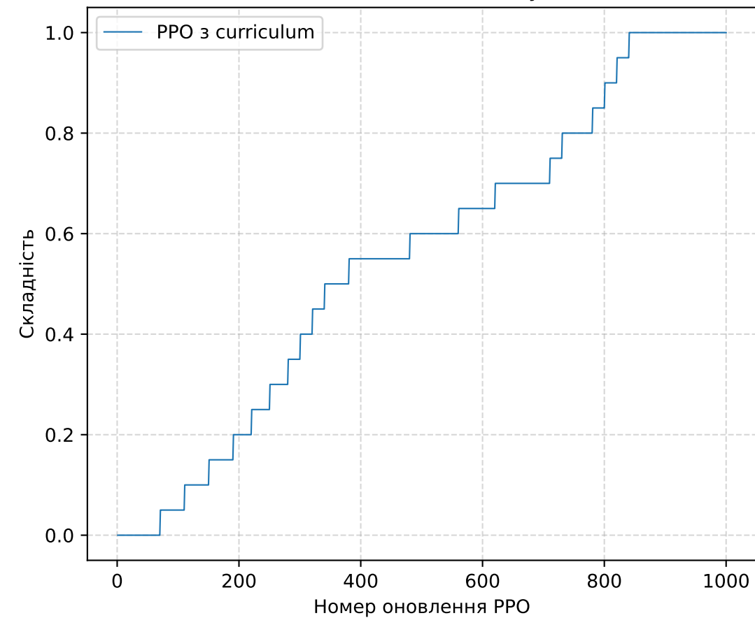
Швидкість навчання
