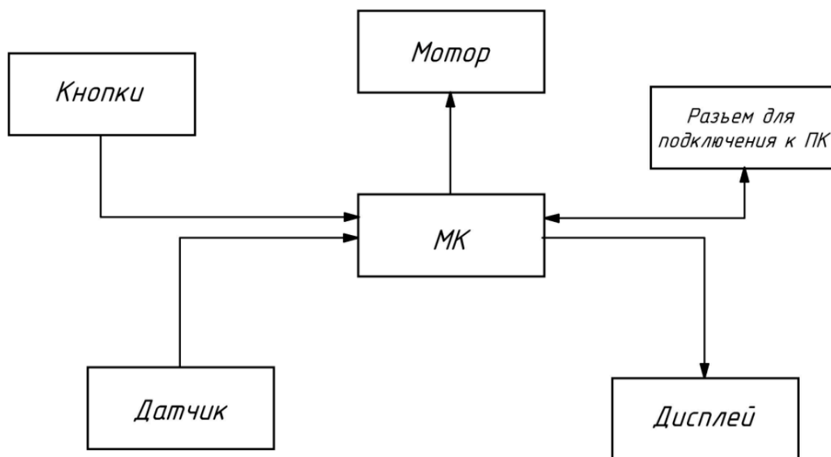
Рисунок 1 — Структурная схема
