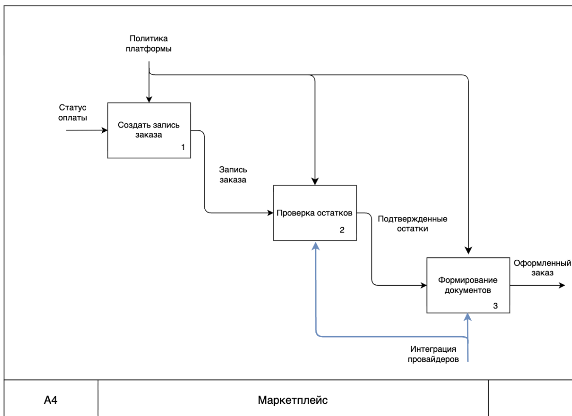
Рисунок 7 — Диаграмма A4 «Регистрация заказа»
