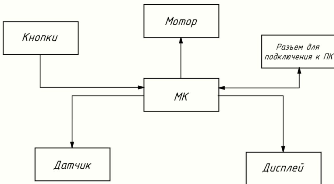
Рисунок 1 — Структурная схема
