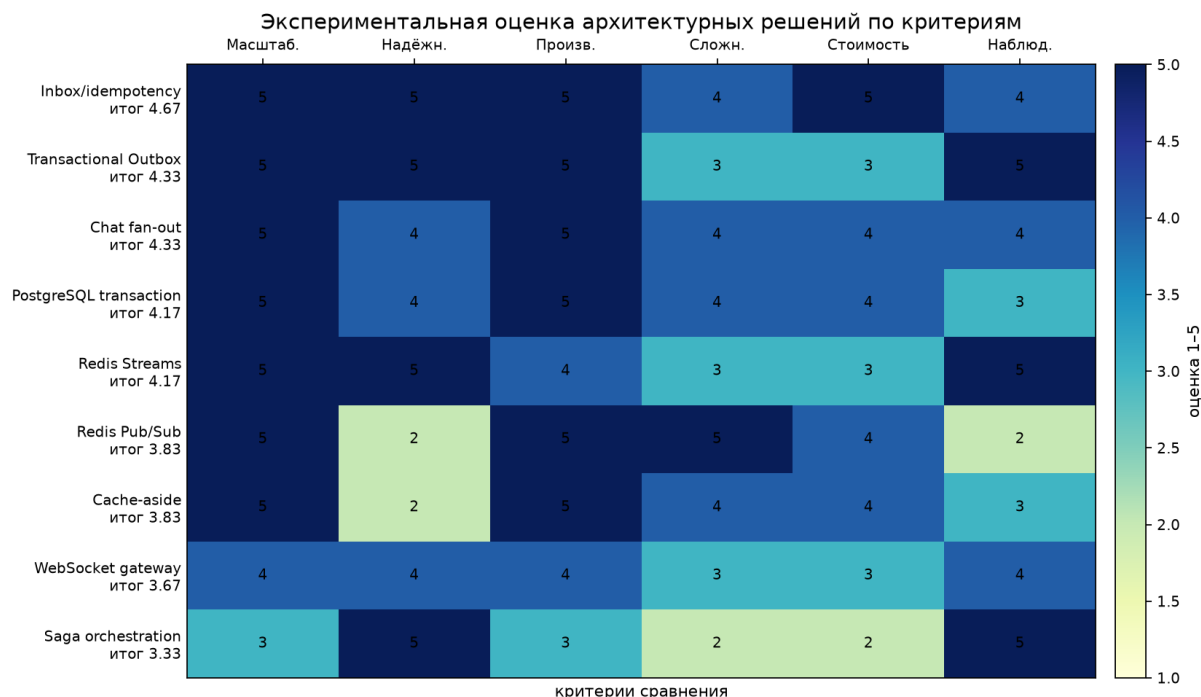
Рисунок 4.4 – Экспериментальная тепловая карта оценок архитектурных компонентов по критериям
