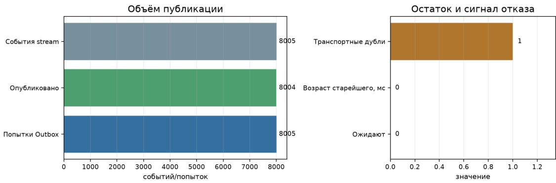
Рисунок 5.2 – Раздельная проверка объёма Outbox/Streams и остаточного backlog
