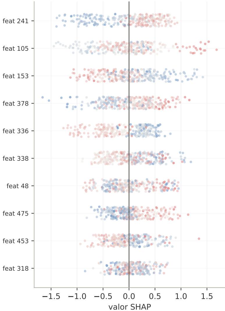
Madelon
