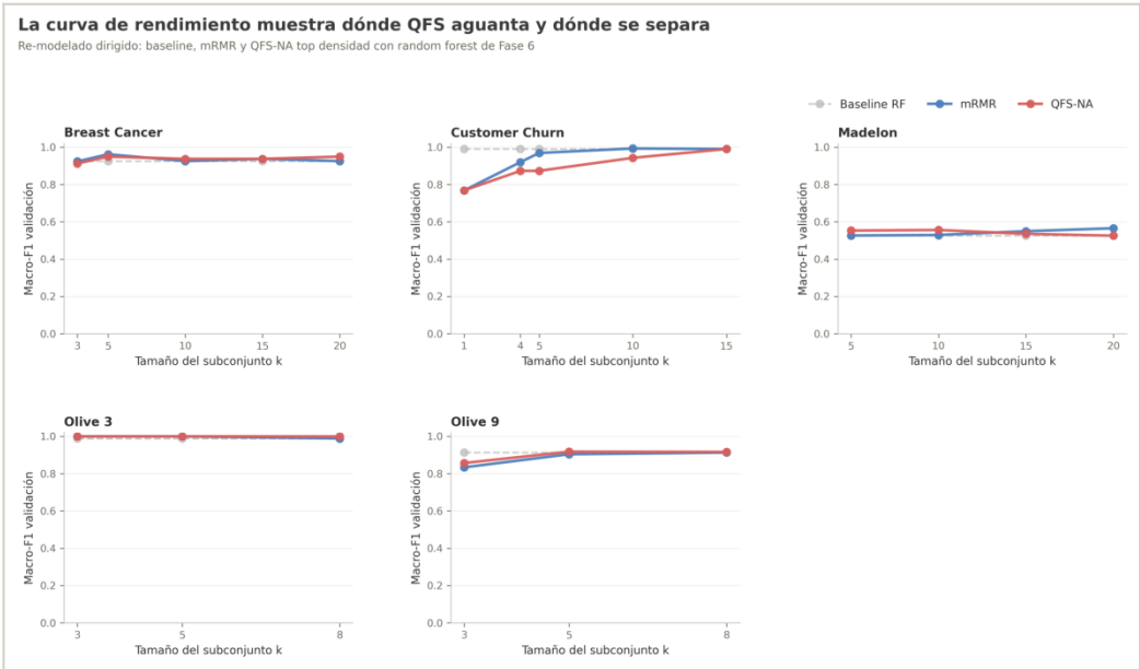
A07 · ev6_rendimiento_vs_k.png
