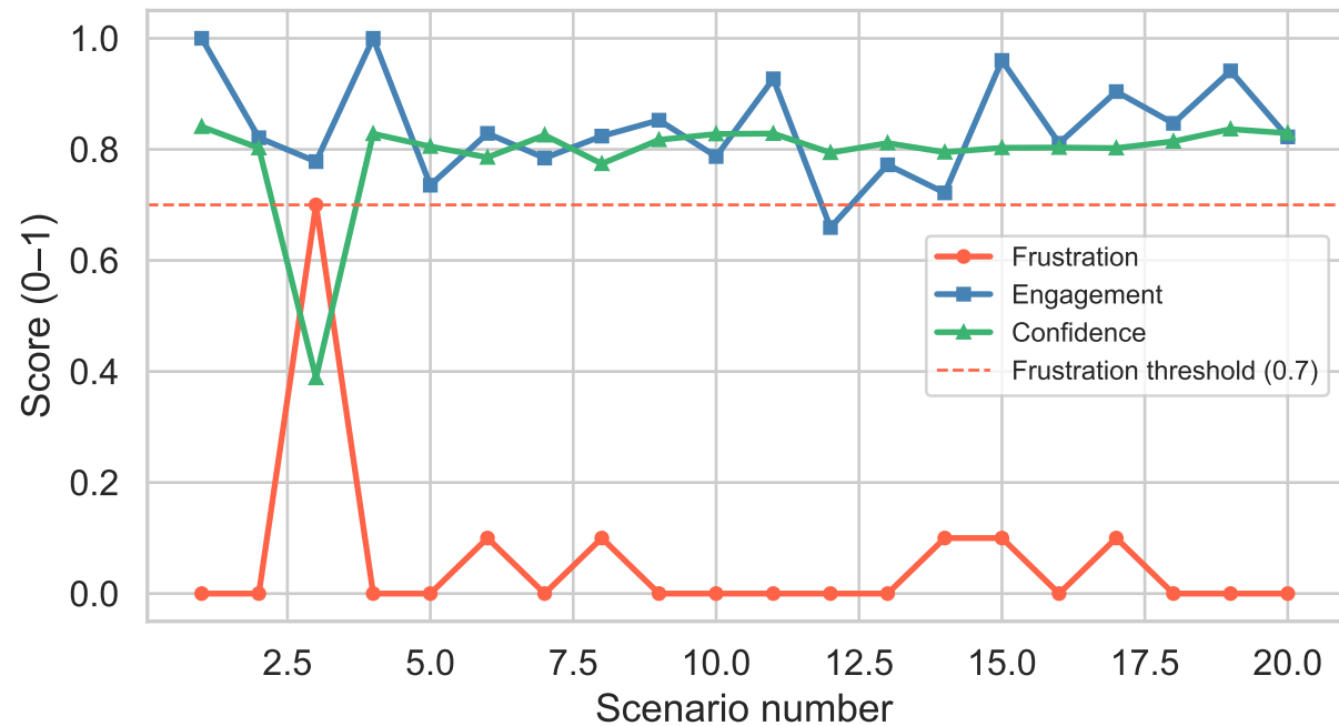
Emotional State Per Scenario
