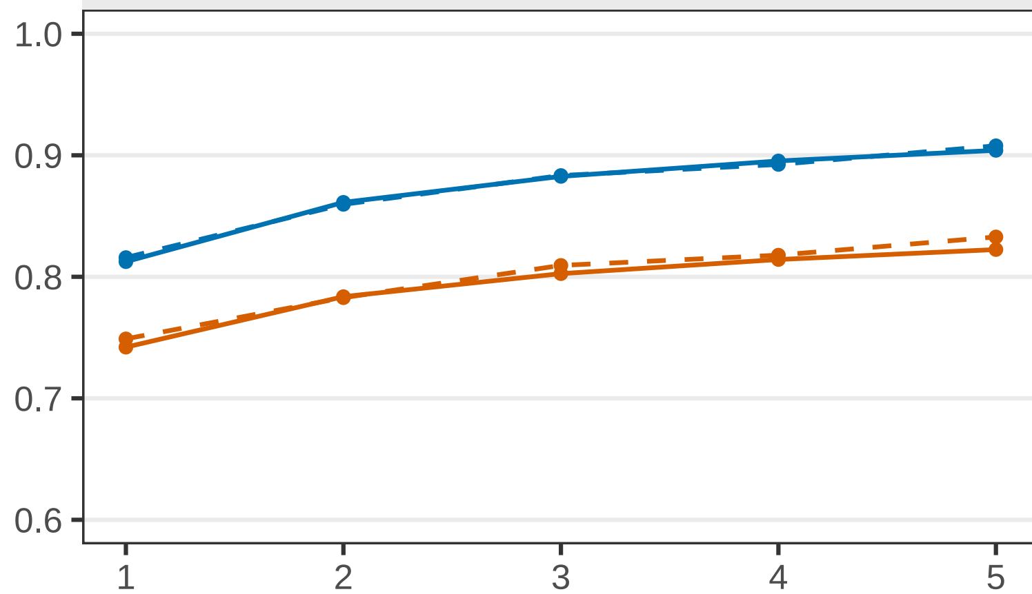
RCP_{H_0} (Method 2)
