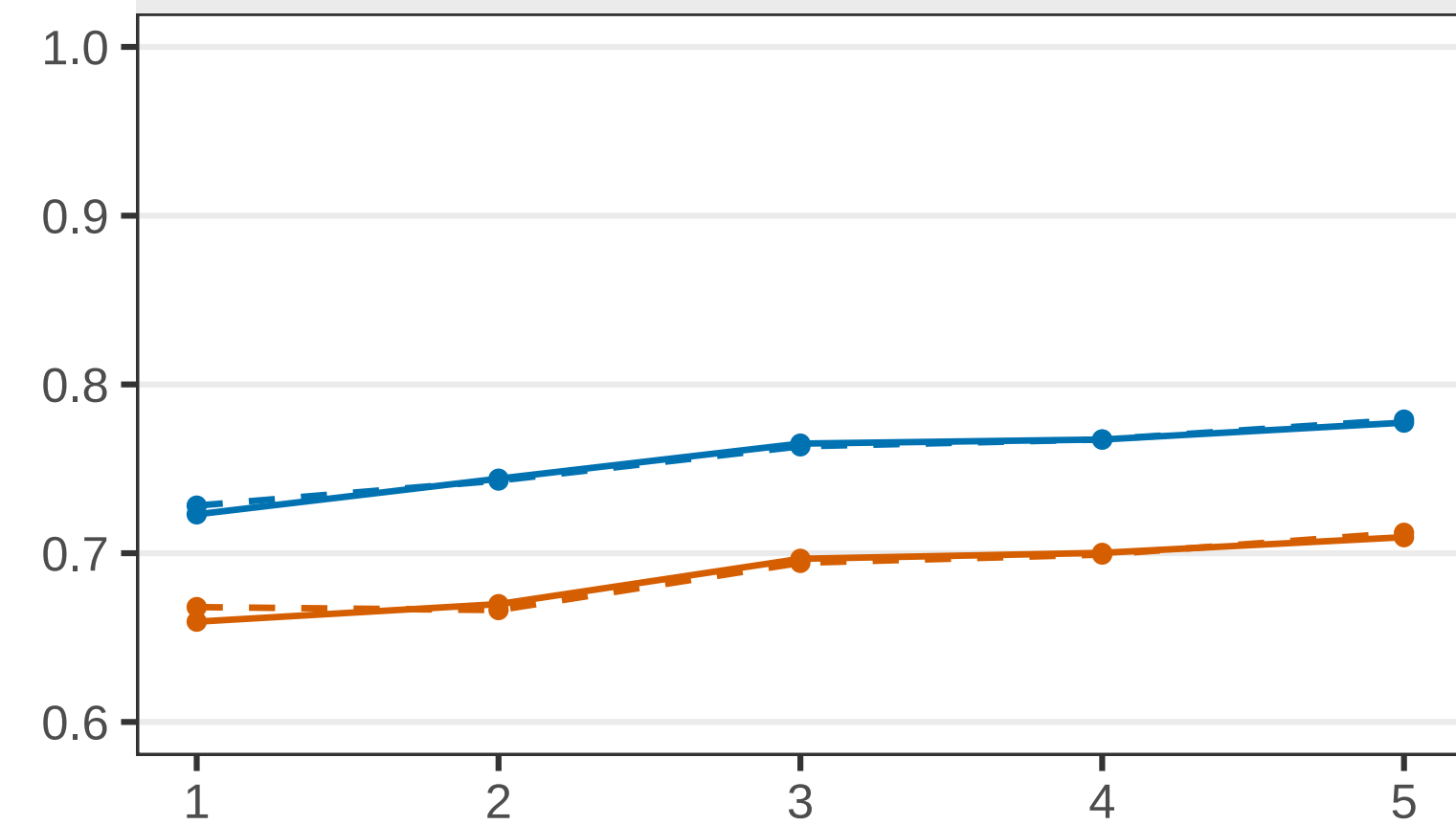
RCP_{H_0} (Method 1)
