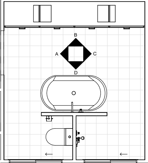
LAYOUT - FF ENS 1 : 50
