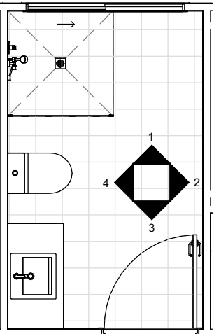
LAYOUT - BATH 1 : 50
