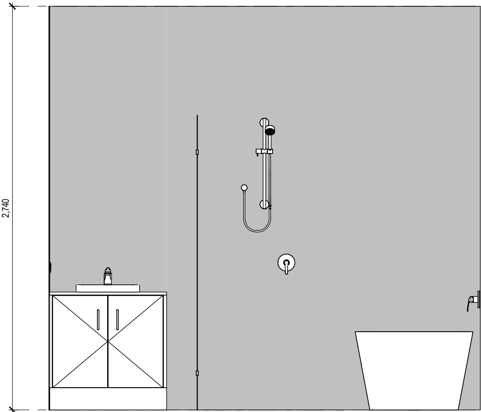
FF BATH A 1 : 25
