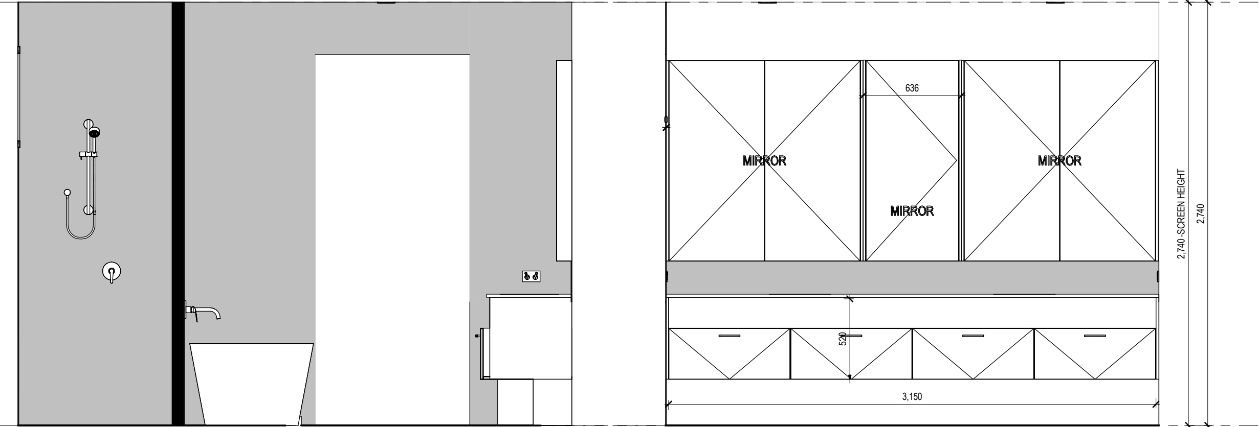
FF ENS A 1 : 25
