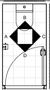
LAYOUT - FF WC 1 : 50
