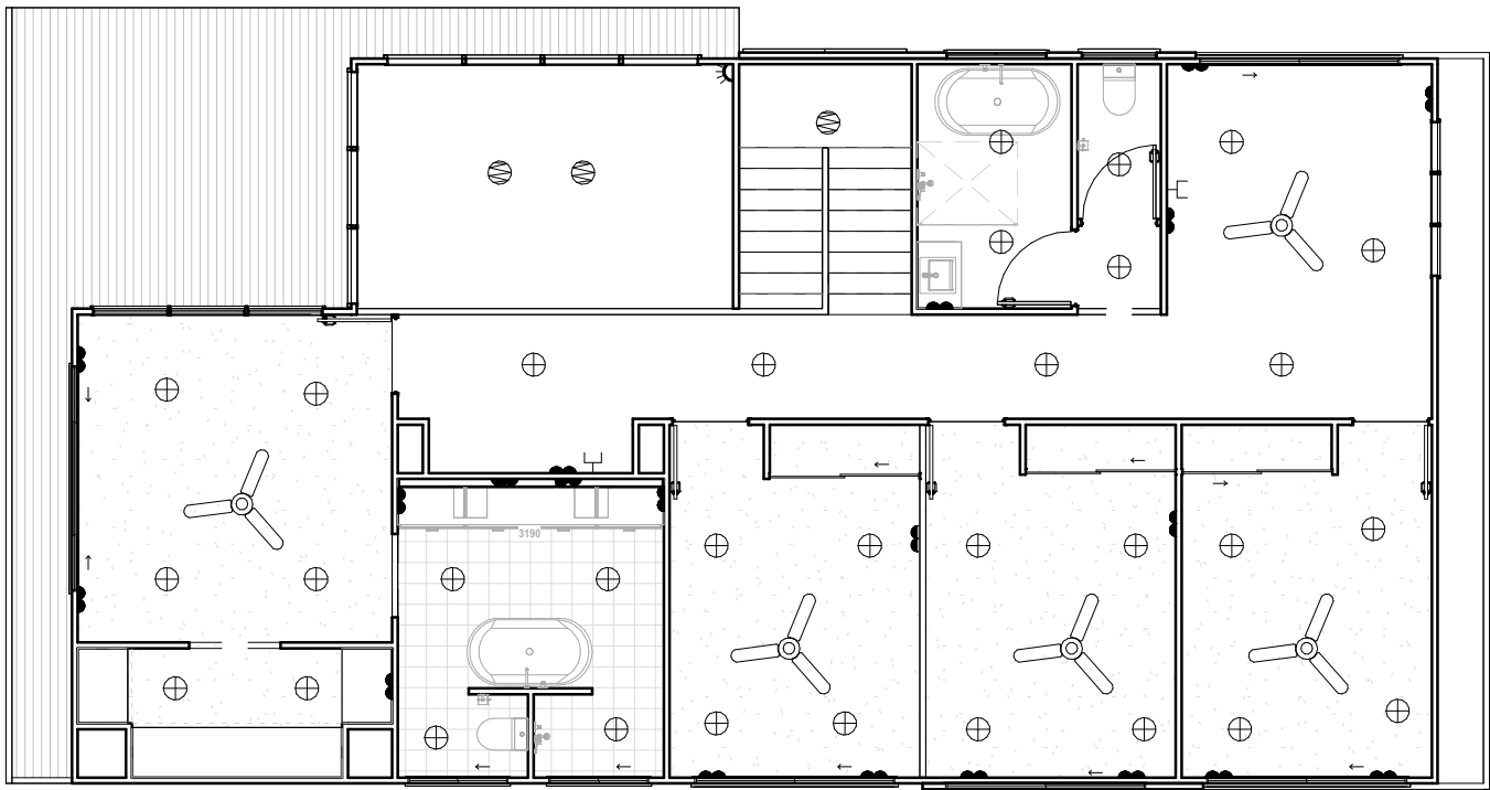
2 FF Electrical Plan 1 : 100
