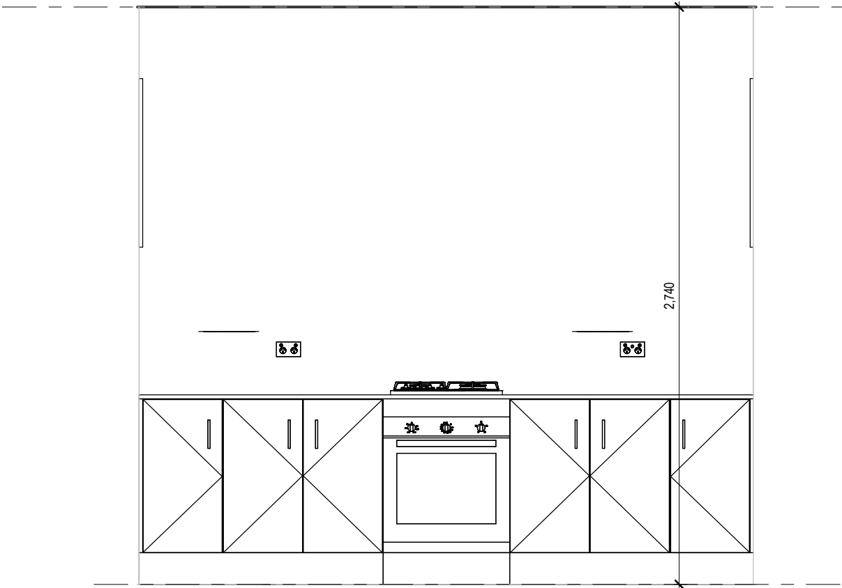
KIT C 1 : 25
