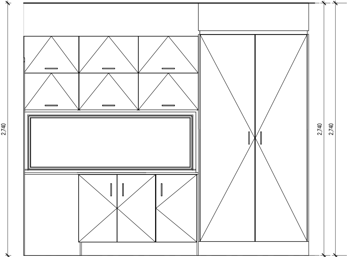
KIT D 1 : 25
