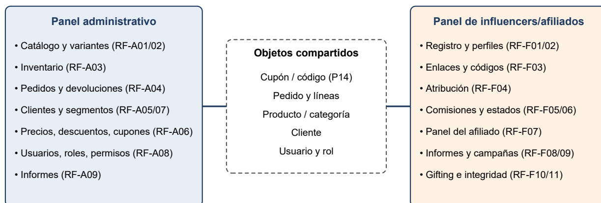
Figura 4. Arquitectura funcional conceptual del sistema propuesto: módulos, requisitos candidatos y objetos compartidos.
