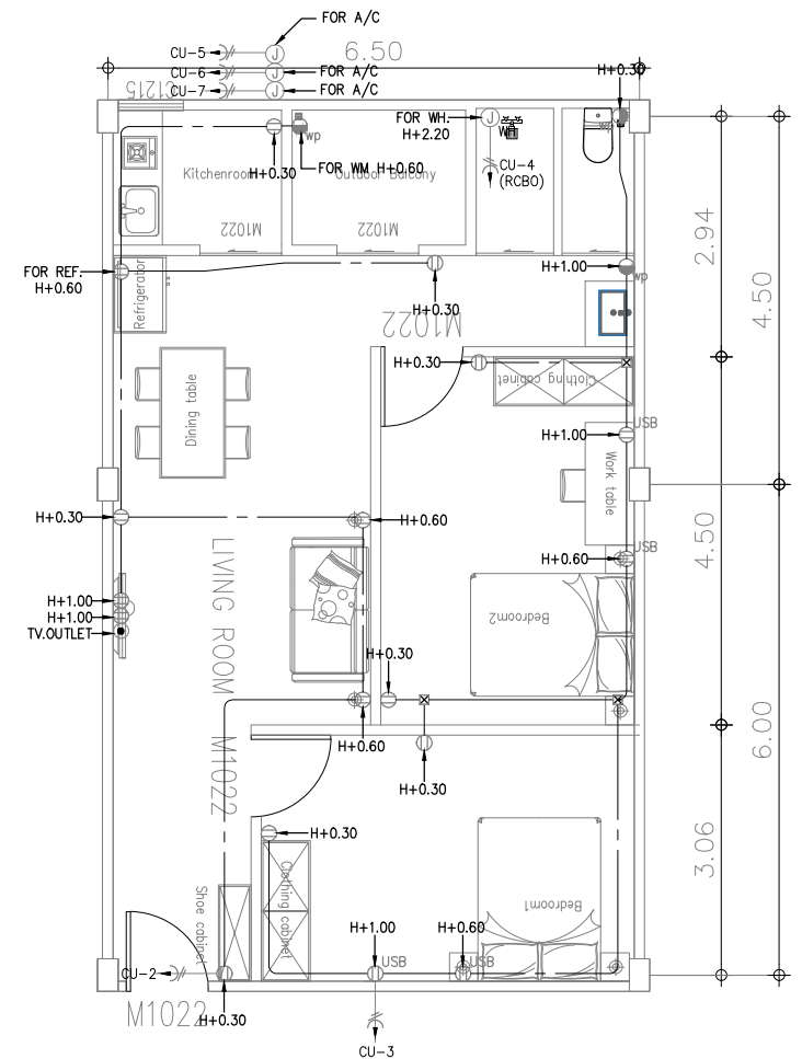
02 แผนระบบเดินไฟฟ้าโทรทัศน์ห้องพัก TYPE B
