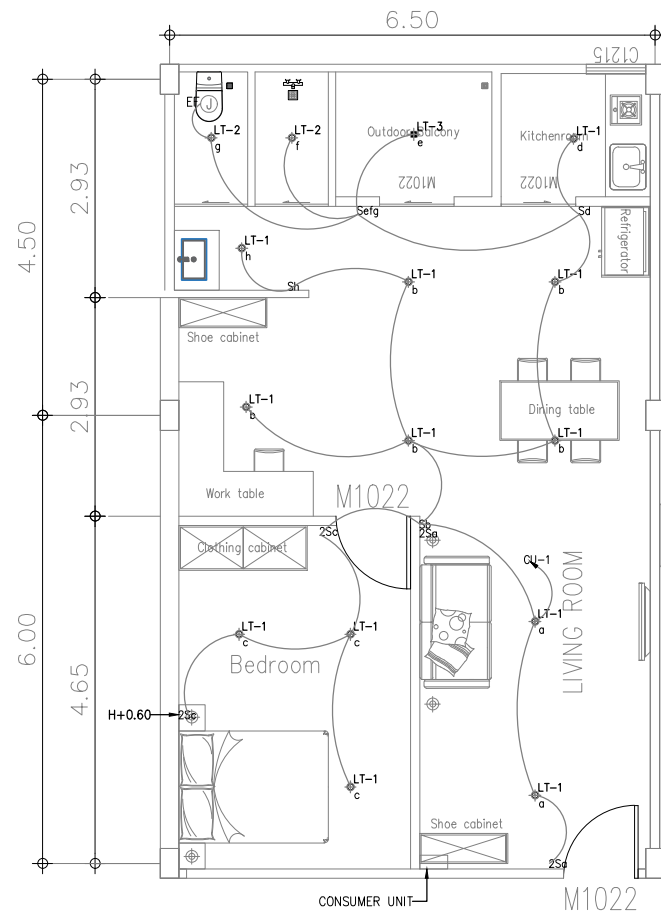
01 แปลนระบบไฟฟ้าแสงสว่างห้องพัก TYPE A
