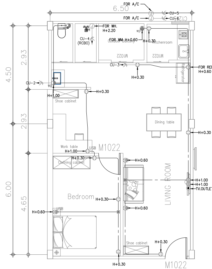
02 แปลนระบบตัวรับไฟฟ้าโทรทัศน์ห้องพัก TYPE A
