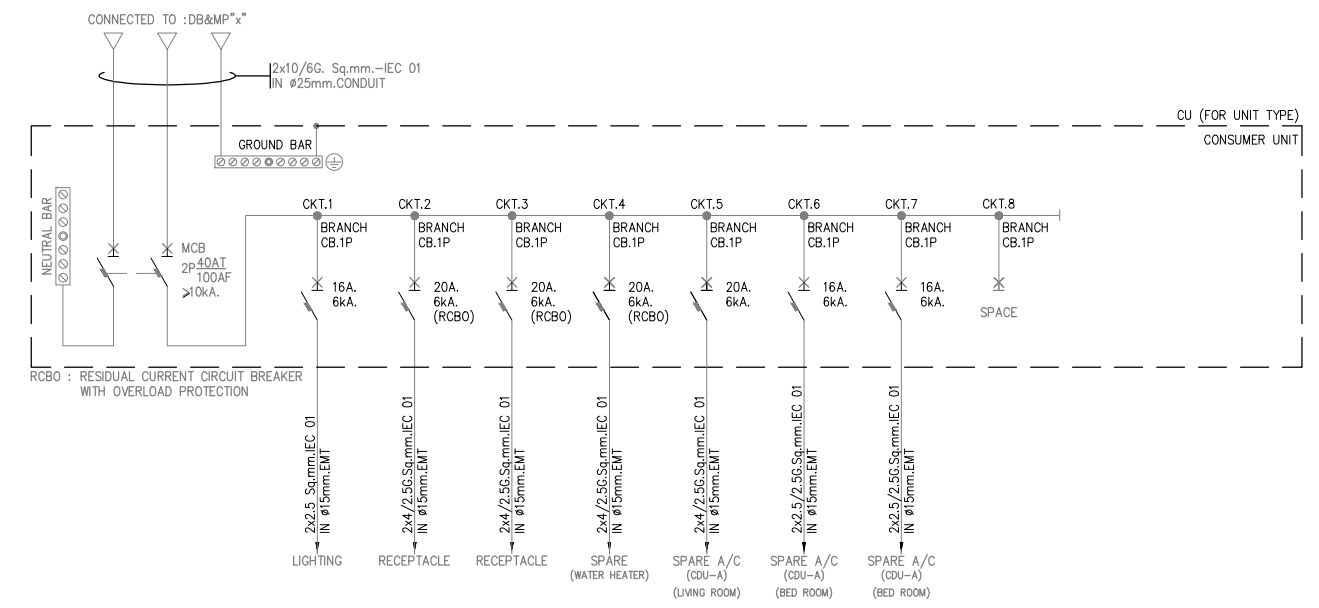
03 ไดอะแกรมเดินด้วยตู้ CU TYPE B
