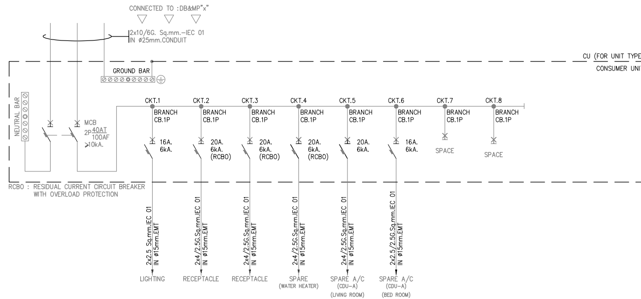
03 ไดอะแกรมเส้นเดียวตัว CU TYPE A NTS
