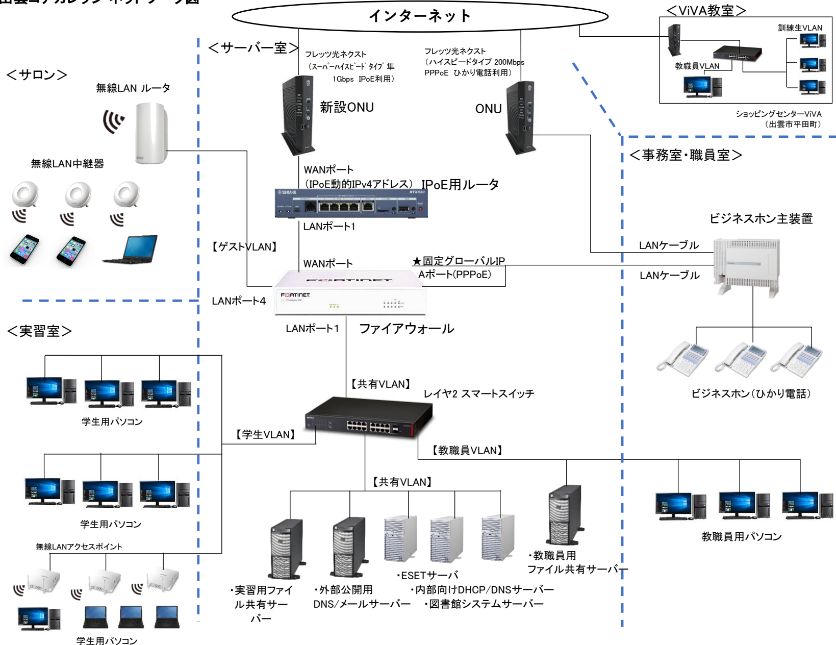
出雲コアカレッジ ネットワーク図
