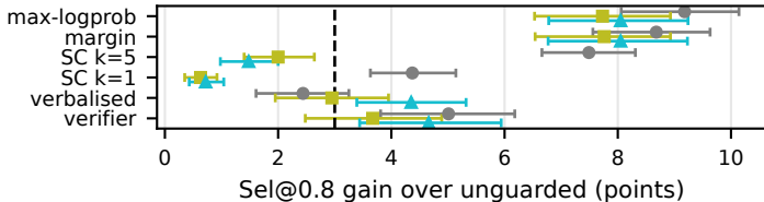
TeleQnA
