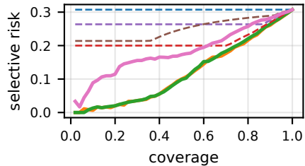
7B
