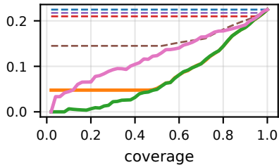
70B
