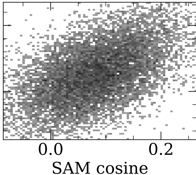
Random (N=10256)
