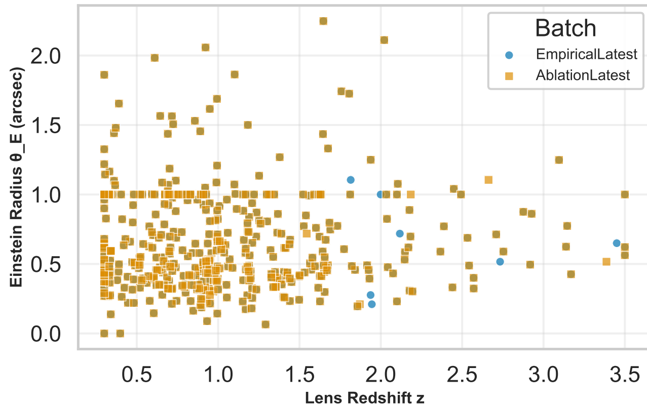
Einstein Radius vs Redshift
