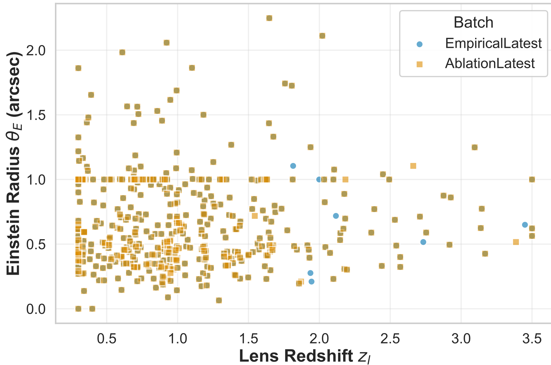
Einstein Radius vs Redshift
