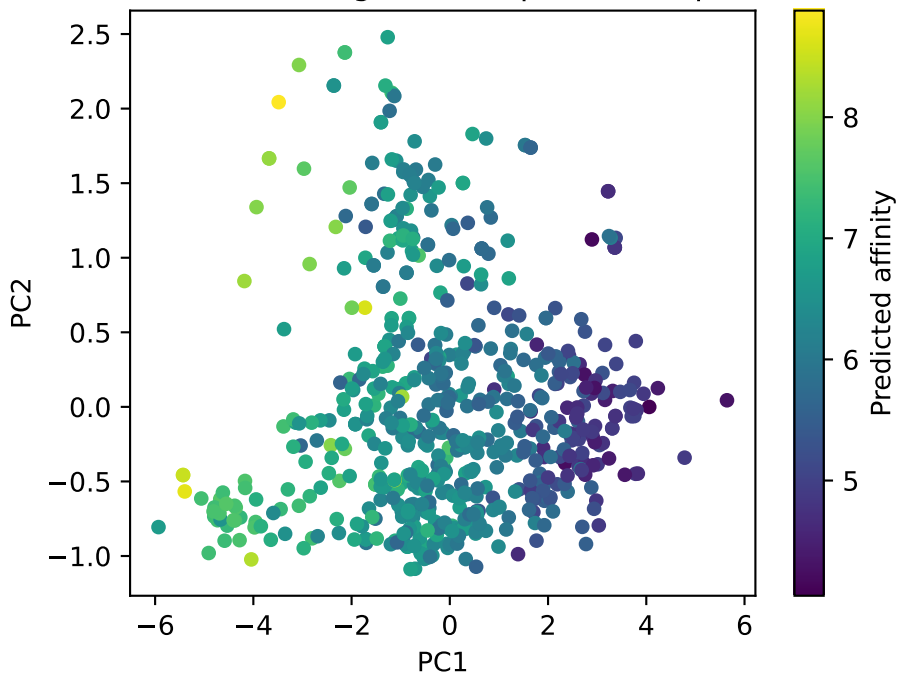
Test embeddings (PCA) - predicted (pna)
