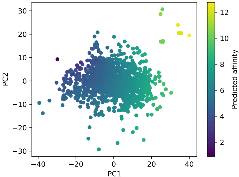
Test embeddings (PCA) - predicted (gin)
