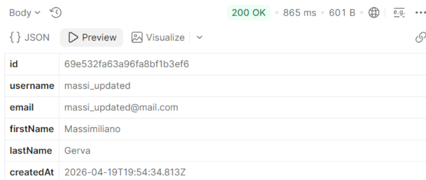
Figura 4.21: Test su Postman: Risposta del server con il profilo aggiornato.
