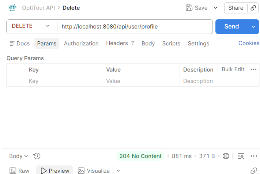
Figura 4.22: Test su Postman: Richiesta di eliminazione dell'account utente.
