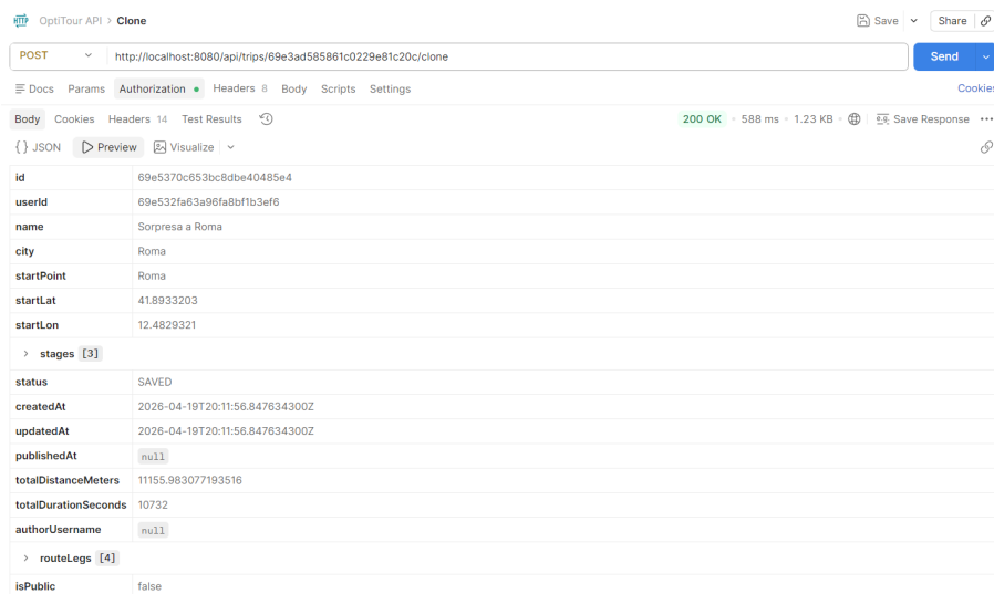
Figura 4.17: Test su Postman: Richiesta di clonazione di un viaggio pubblico.
