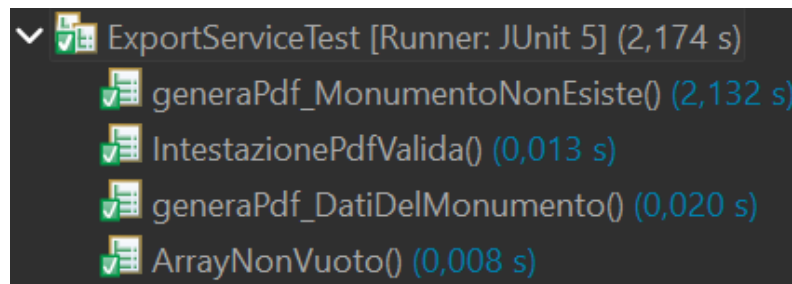
Figura 4.12: Test classe "ExportService" per gestione dell'esportazione del viaggio
