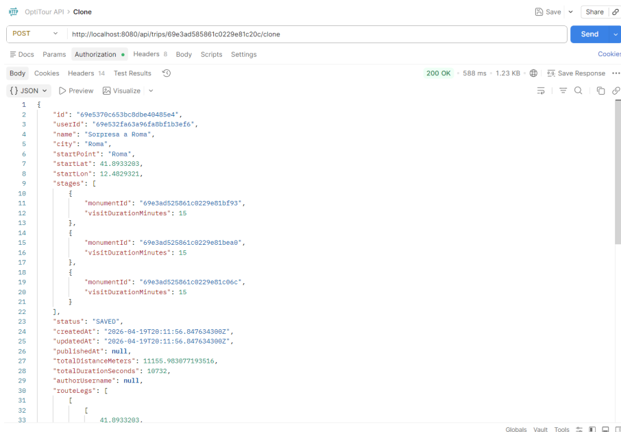
Figura 4.18: Test su Postman: Risposta del server con il viaggio clonato.
