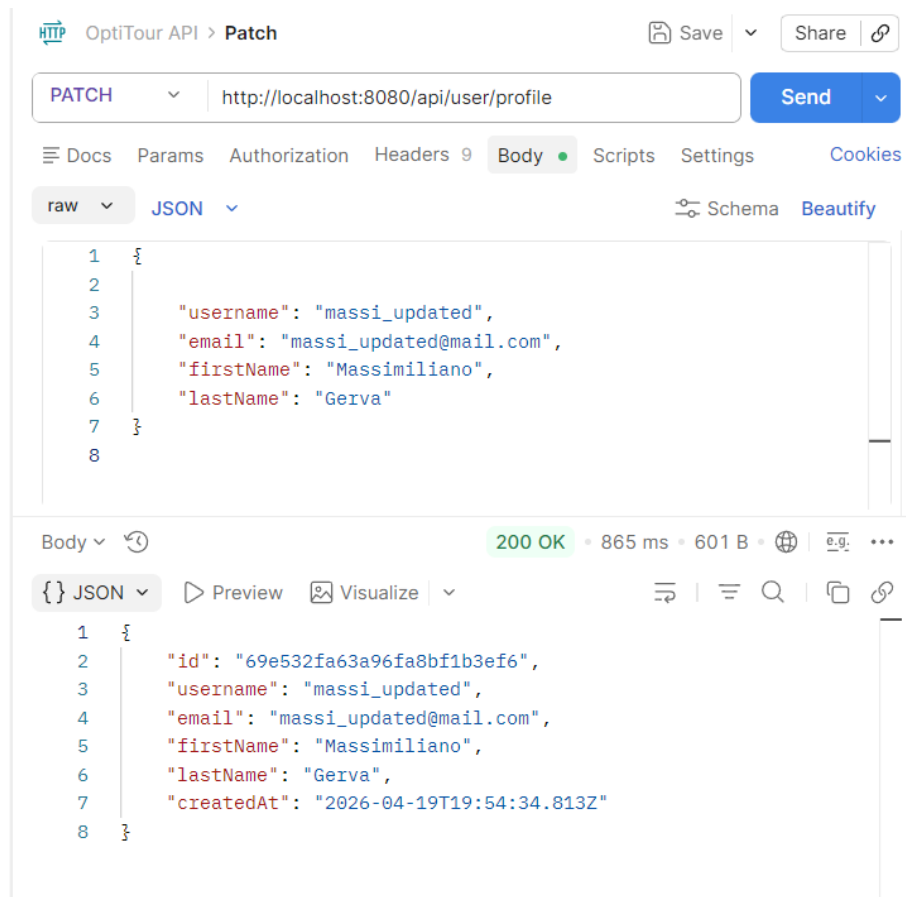
Figura 4.20: Test su Postman: Payload di richiesta per l'aggiornamento del profilo utente.
