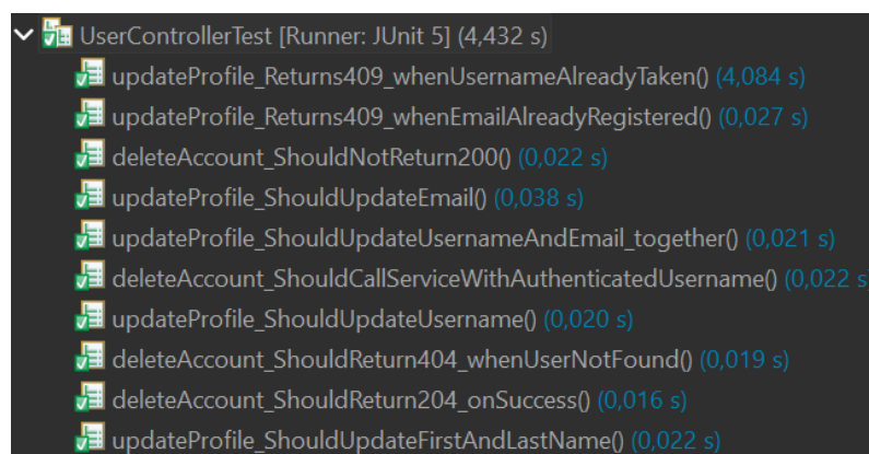
Figura 4.10: Test classe "UserController" per gestione profilo utente
