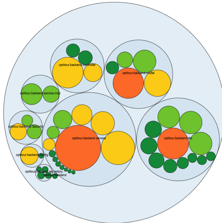
Figura 4.9: Distribuzione delle metriche all'interno dei package.
