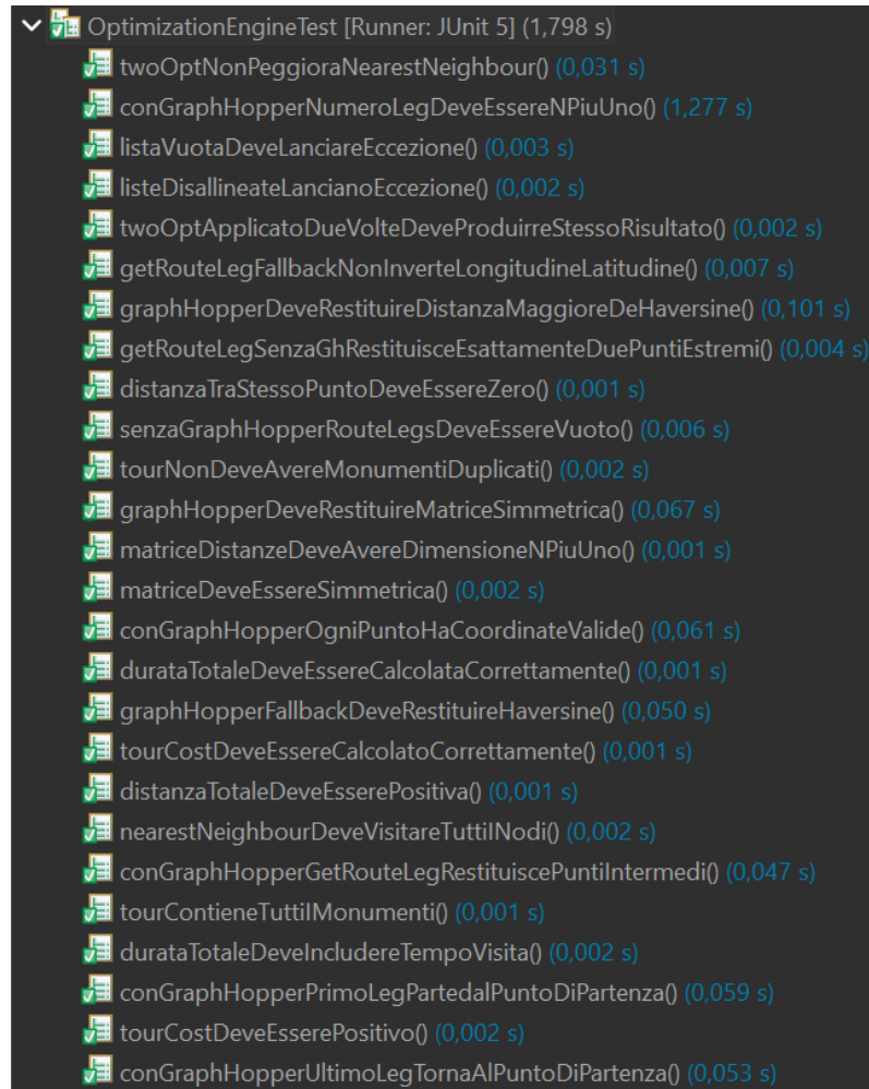
Figura 4.14: Test classe "OptimizationEngine" per l'ottimizzazione del percorso
