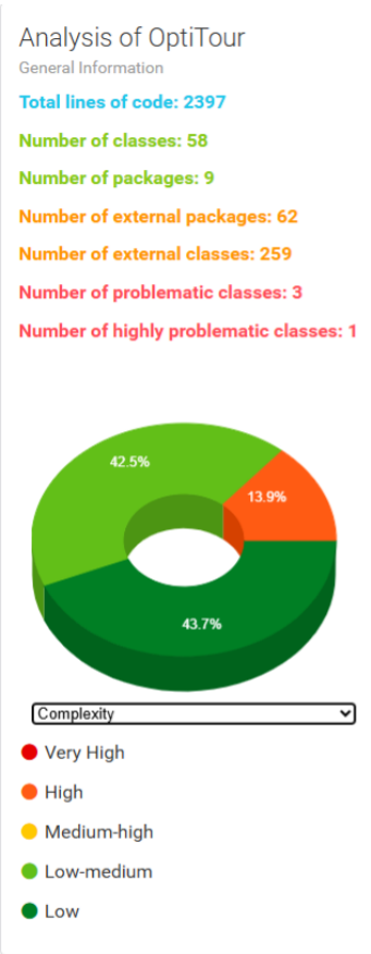
Figura 4.3: Complessità.
