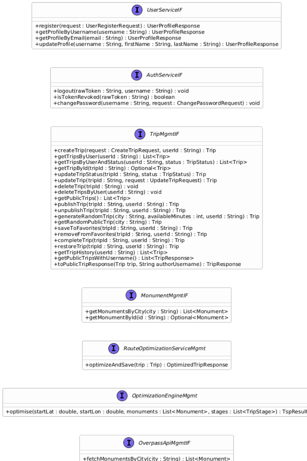
Figura 3.1: Diagramma delle interfacce - Iterazione 2.
