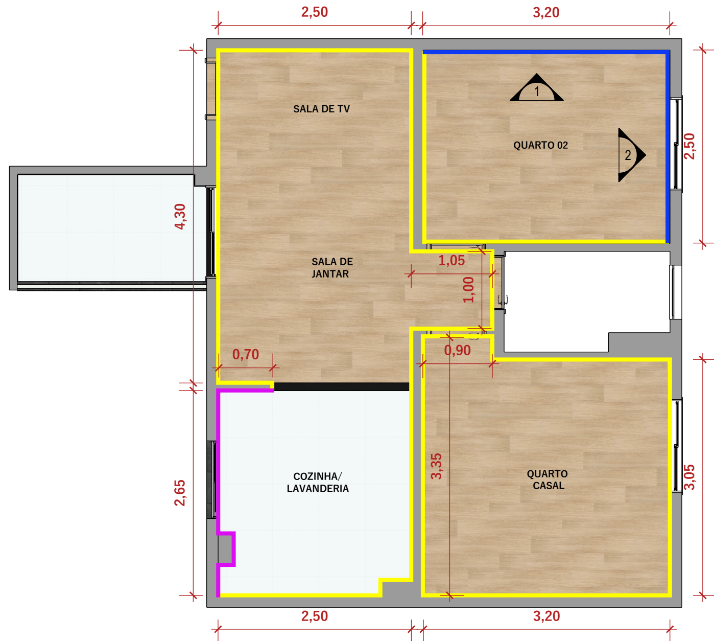
PLANTA BAIXA - ACABAMENTOS ESC 1:50
