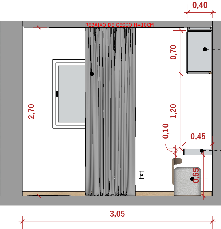
09 VISTA 09 ESC 1:35
