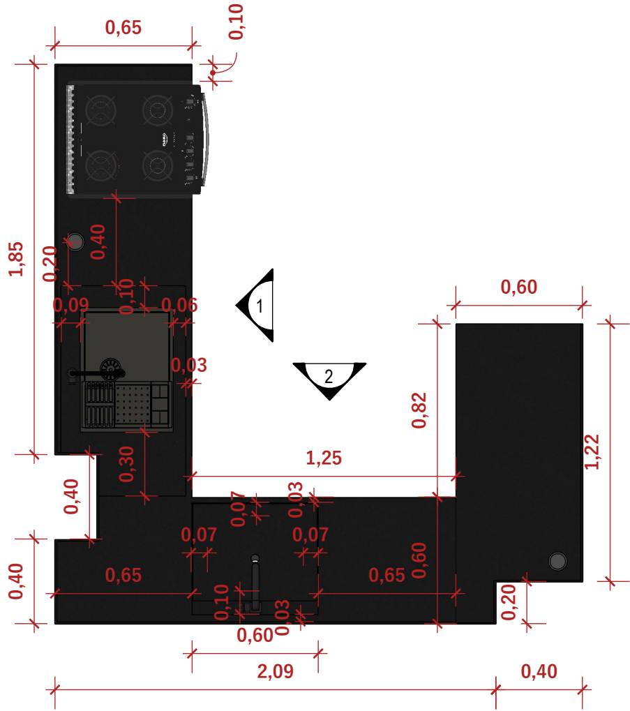
PLANTA BAIXA - BANCADA ESC 1:25
