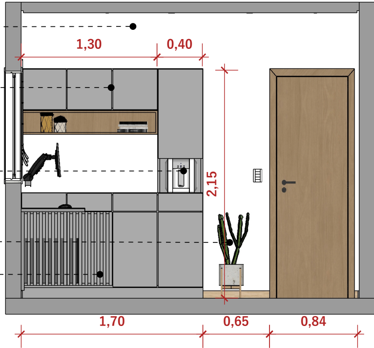
14 VISTA 14 ESC 1:35
