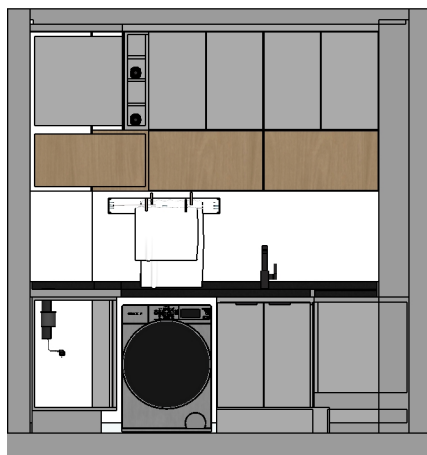
07 VISTA 07 ESC 1:50
