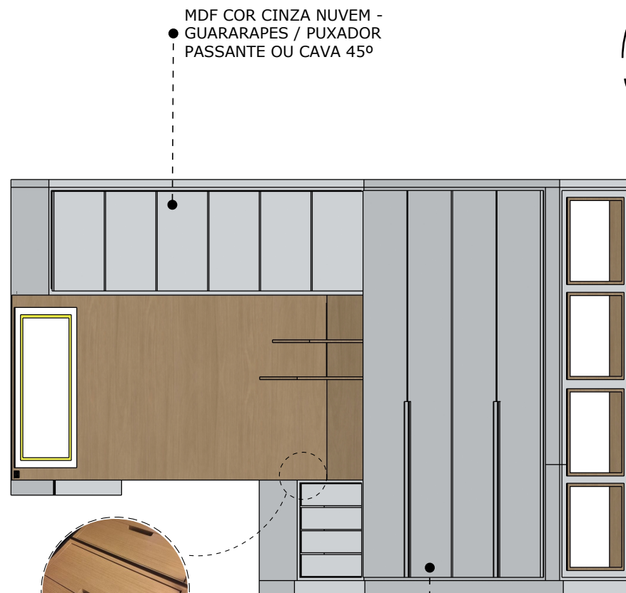
10 VISTA 10 ESC 1:35
