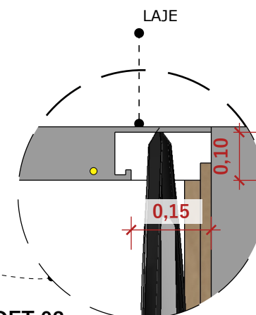
DET 02: ESCALA 1:10 CORTINA COM TRILHO SUÍÇO
