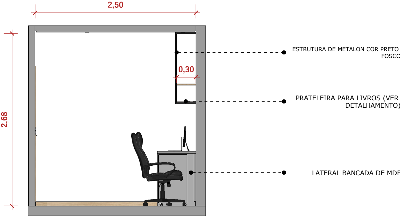
15 VISTA 15 ESC 1:35
