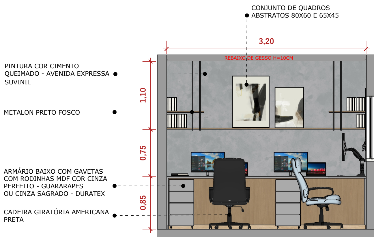
12 VISTA 12 ESC 1:35
