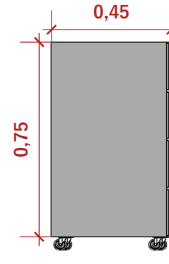
VISTA LATERAL - GAVETAS ESC 1:20
