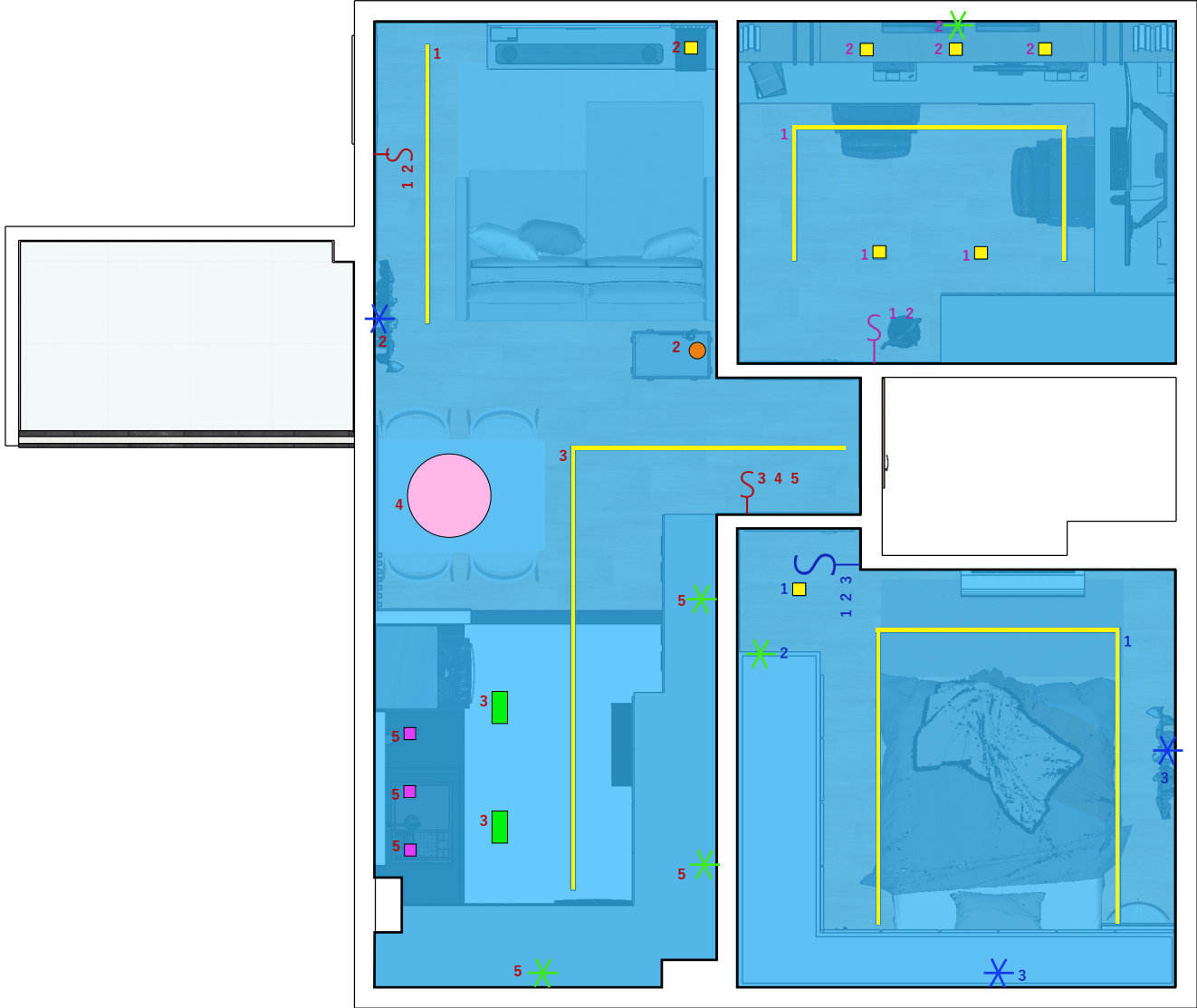
PLANTA CIRCUÍTO ESC 1:50
