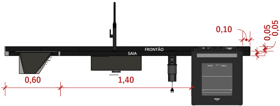
VISTA FRONTAL 01 ESC 1:25
