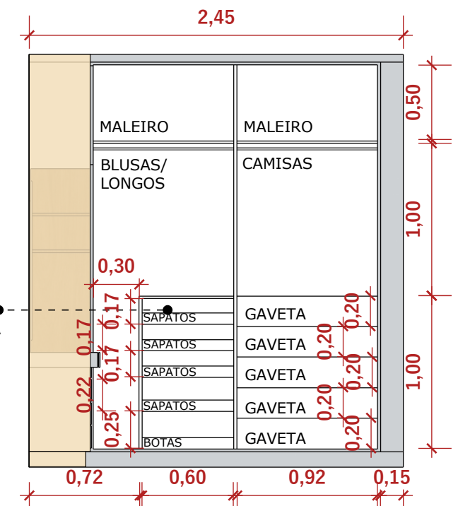
VISTA FRONTAL GUARDA-ROUPA ABERTO ESCALA 1:35
