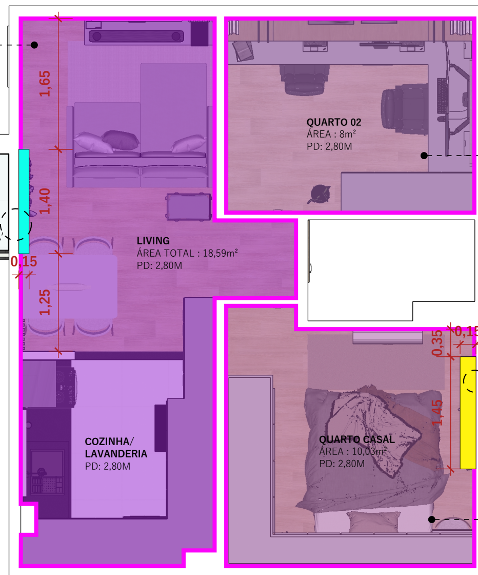
PLANTA DE GESSO ESC 1:50
