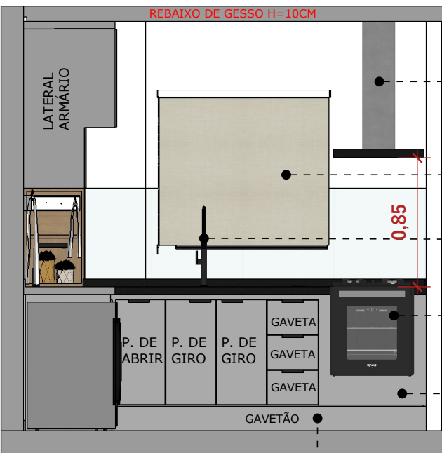
05 VISTA 05 ESC 1:35
