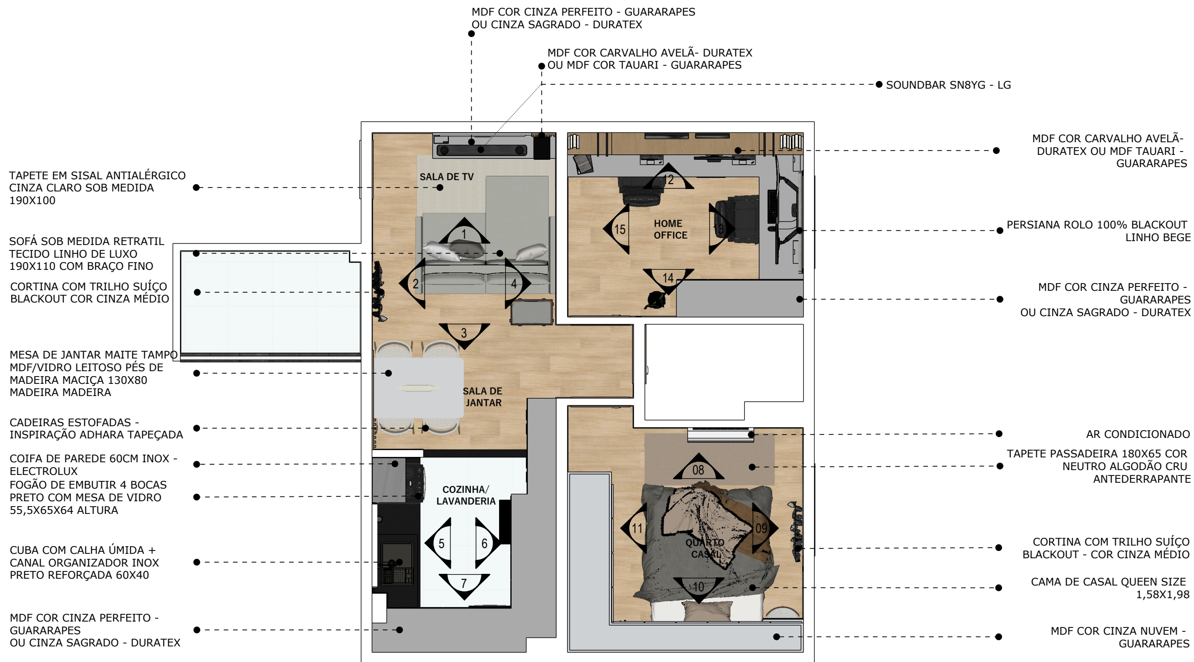
01 PLANTA DE LAYOUT ESC 1:50
