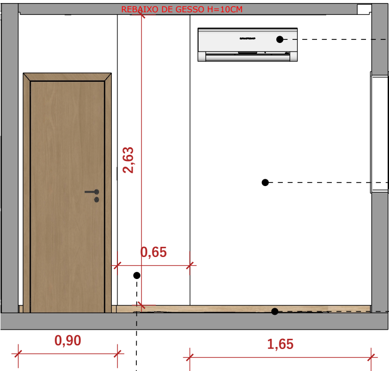
08 VISTA 08 ESC 1:35
