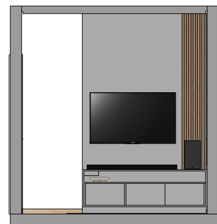
01 VISTA 01 ESC 1:50
