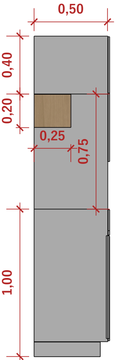
VISTA LATERAL - ARMÁRIO ESC 1:25
