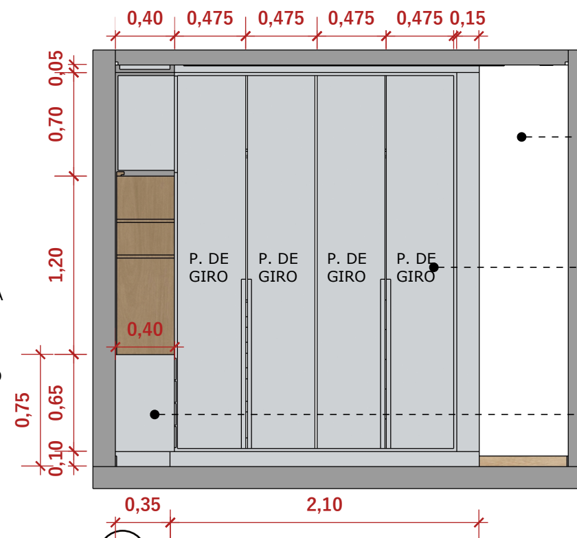
11 VISTA 11 ESC 1:35
