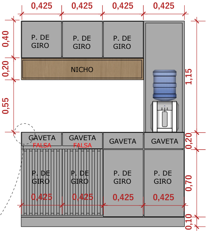
VISTA FRONTAL - ARMÁRIO HOME OFFICE ESC 1:25
