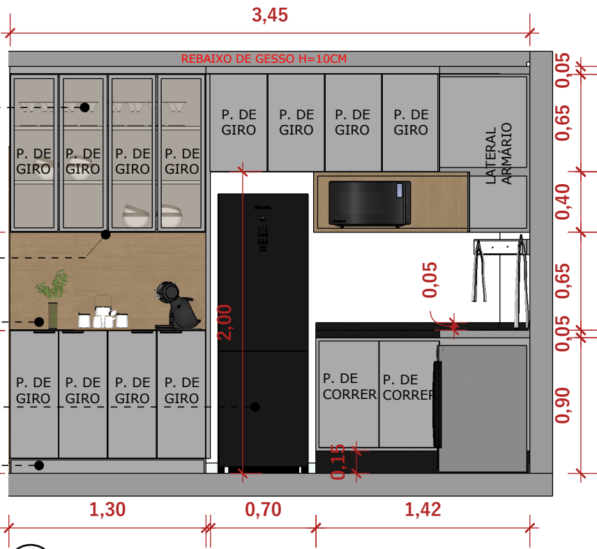
06 VISTA 06 ESC 1:35
