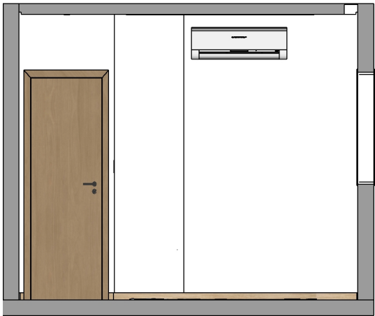
08 VISTA 08 ESC 1:50
