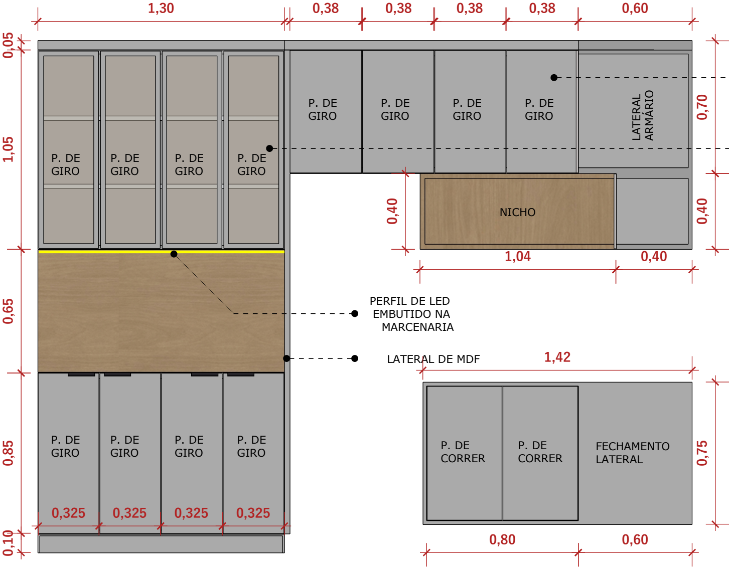
VISTA A ESC 1:20
