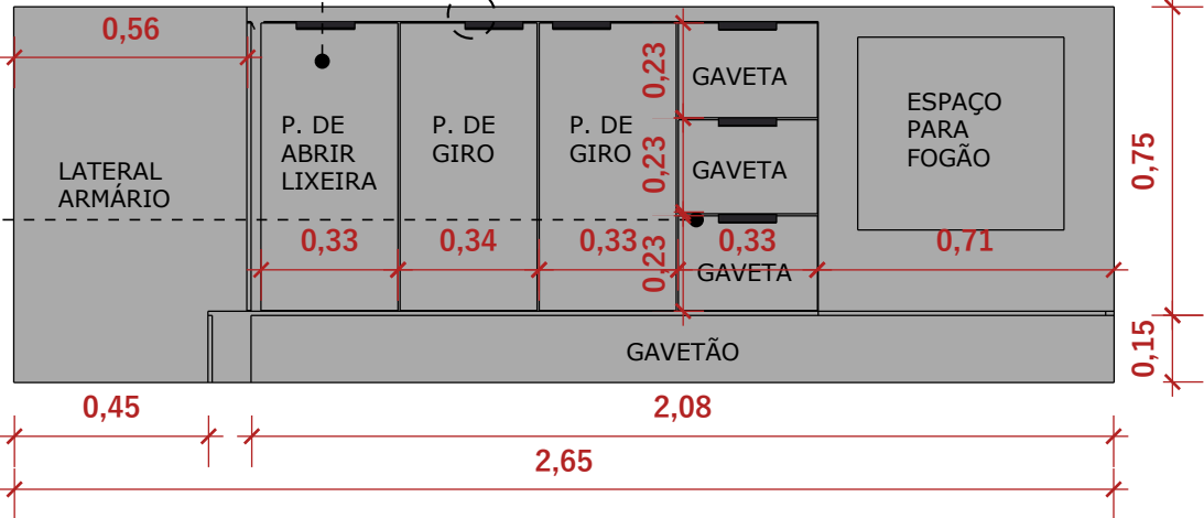
VISTA B ESC 1:20
