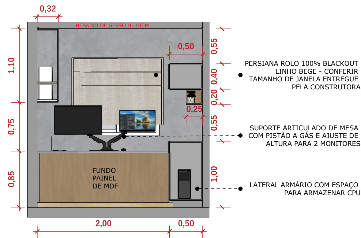
13 VISTA 13 ESC 1:35
