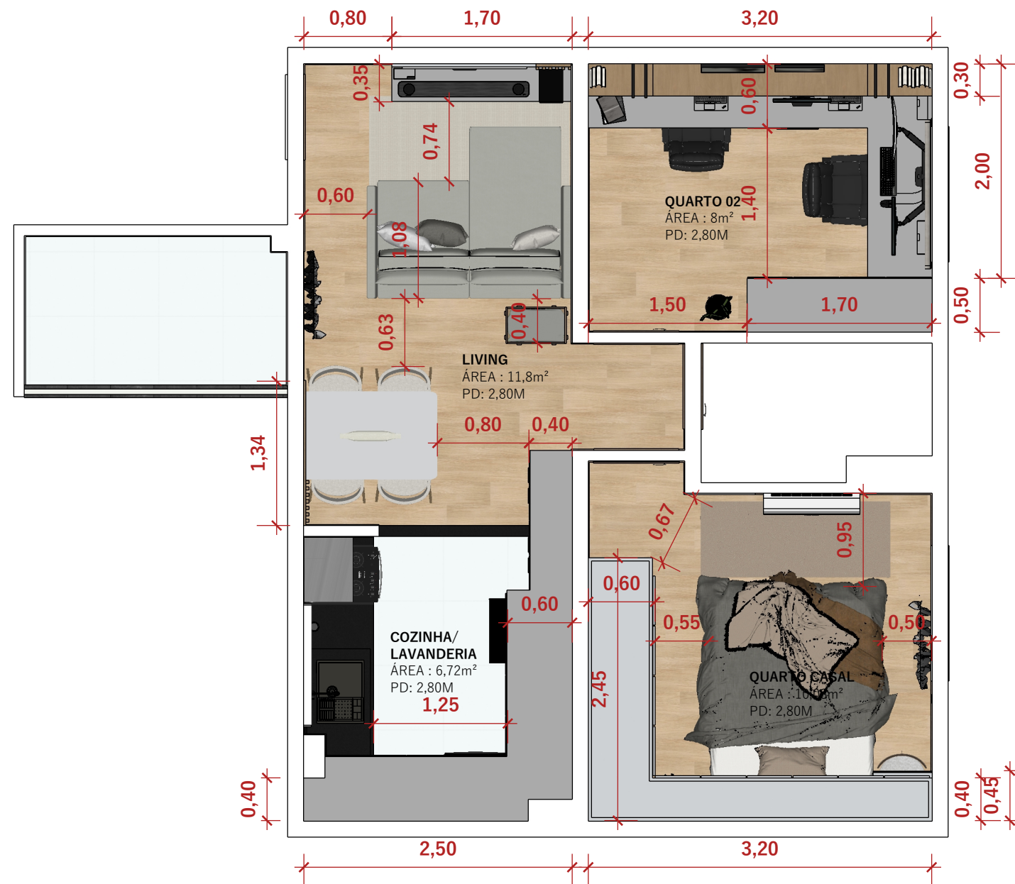
PLANTA BAIXA EXECUTIVA ESC 1:50
