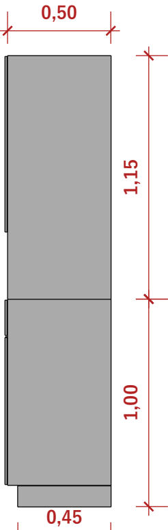
VISTA LATERAL - ARMÁRIO ESC 1:25
