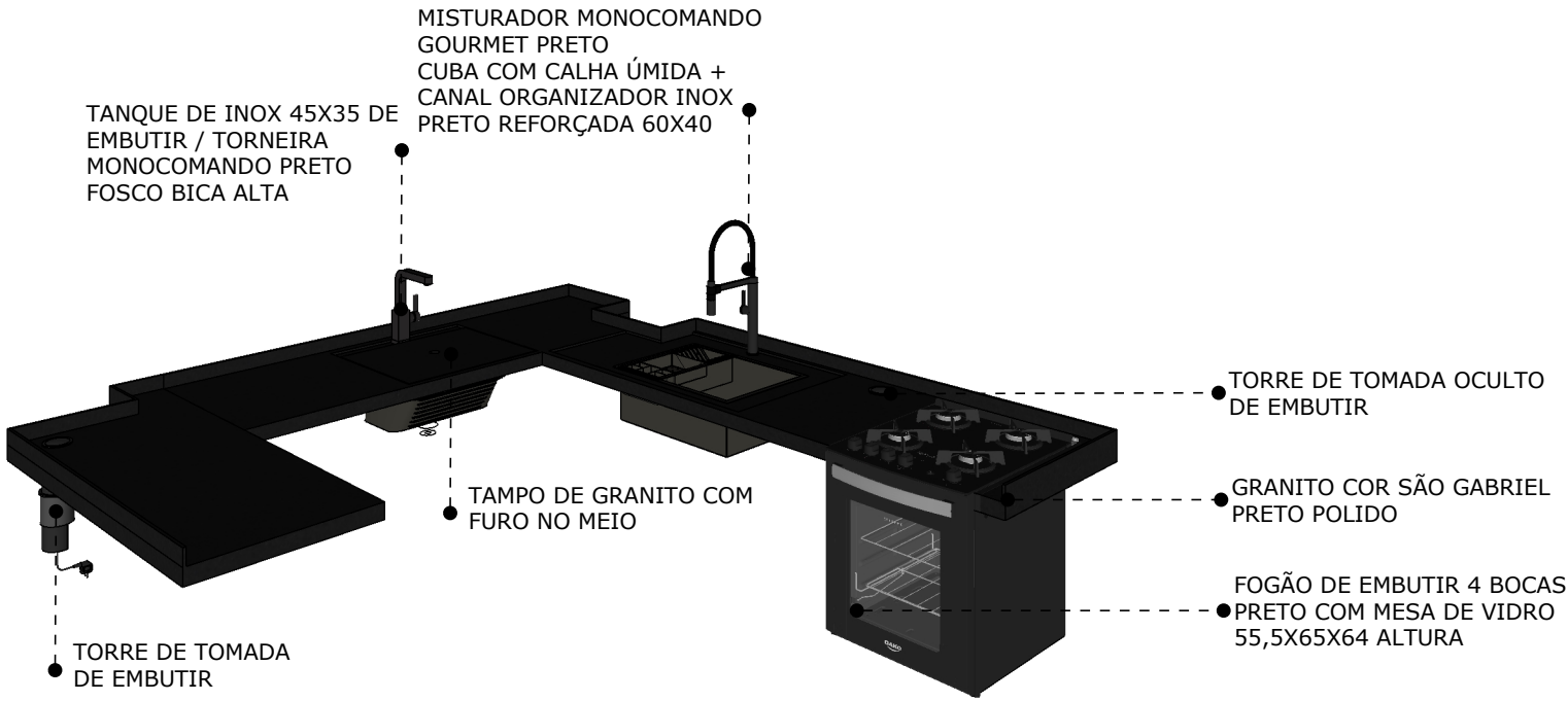
PERSPECTIVA - PIA E TANQUE SEM ESCALA
