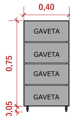
VISTA FRONTAL - GAVETAS ESC 1:20
