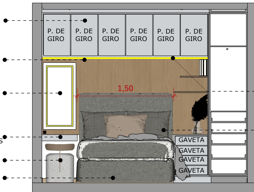
10 VISTA 10 ESC 1:35
