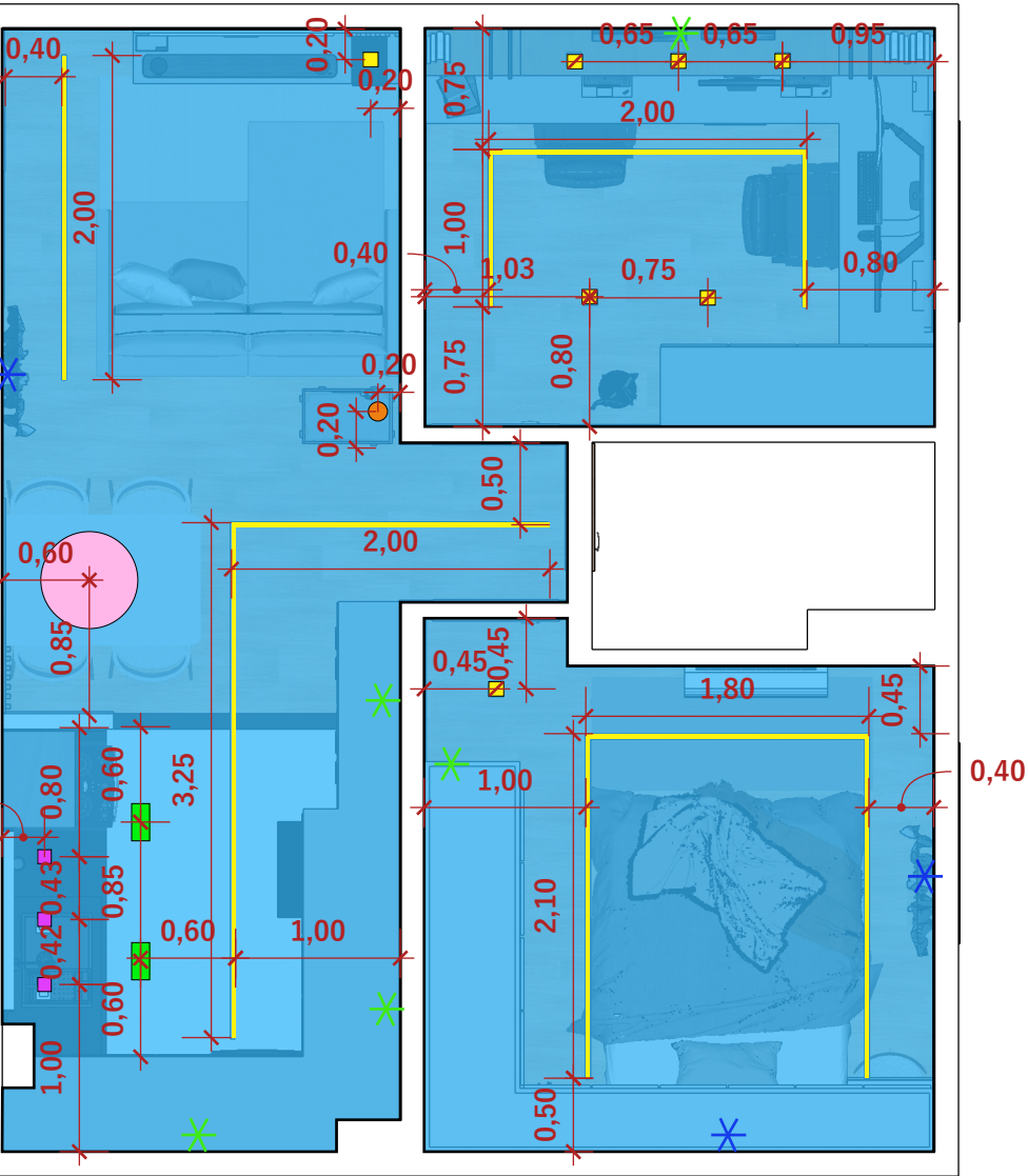
PLANTA LUMINOTÉCNICA ESC 1:50
