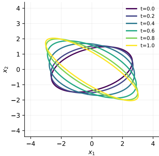
cosine
