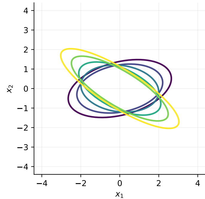
linear
