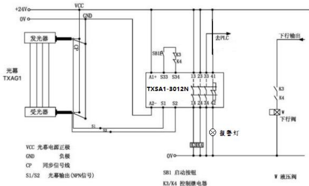
接线图
