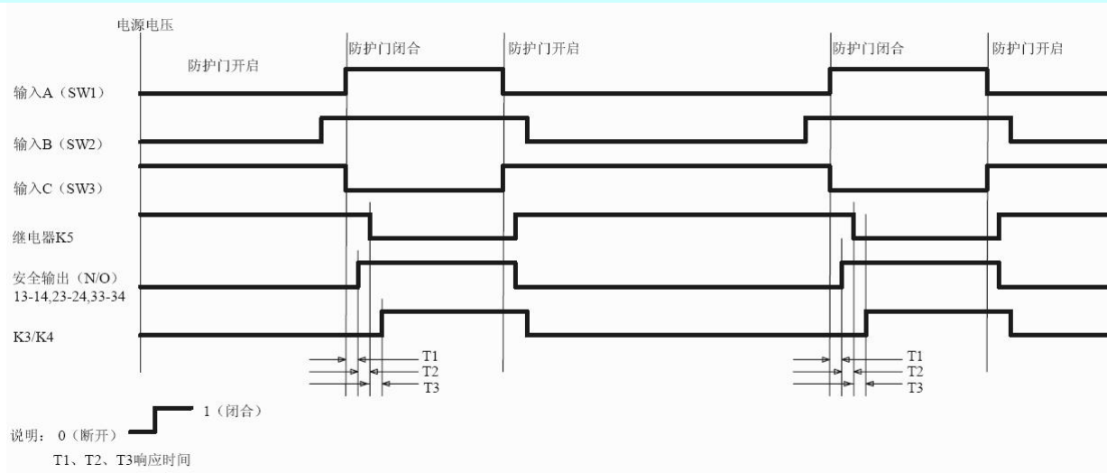
时序图
