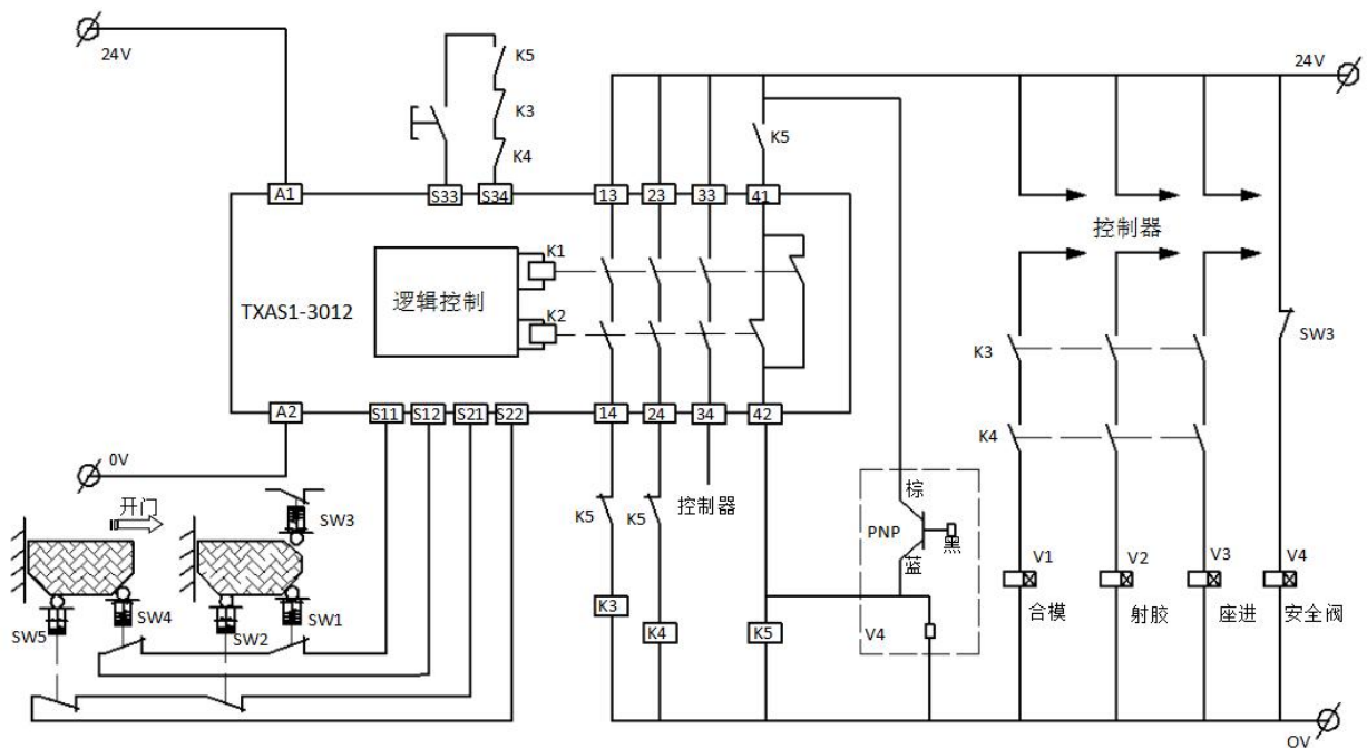
接线图
