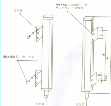
通用L型支架安装方式
