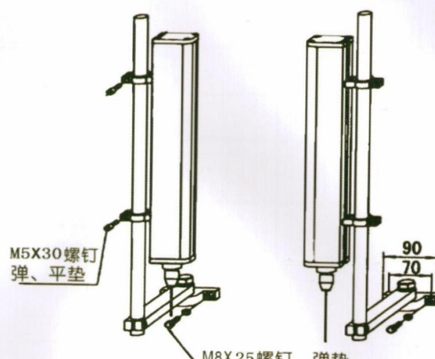
钢管活动支架安装方式
