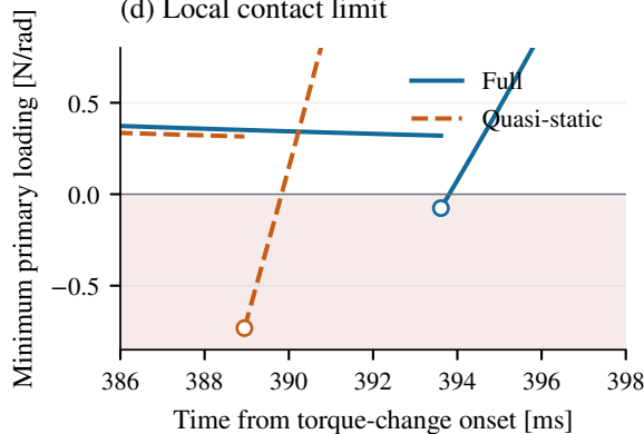
(d) Local contact limit
