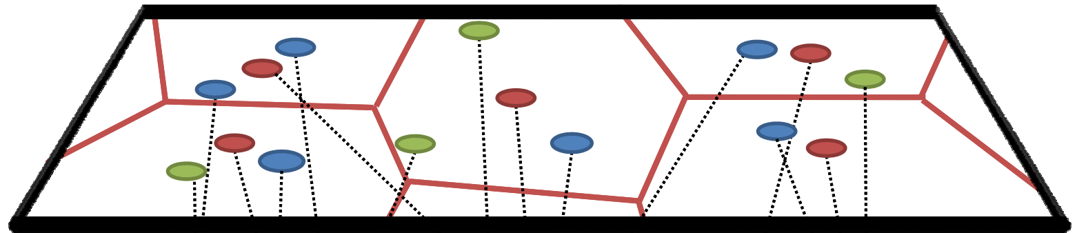
RayNet Layer
