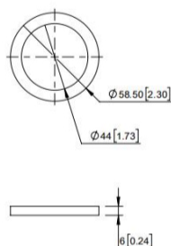
Fig 4 : Gasket
