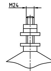
380V,400V,420V 套管接线端子
