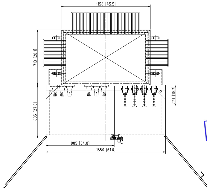
L.V. TERMINAL
