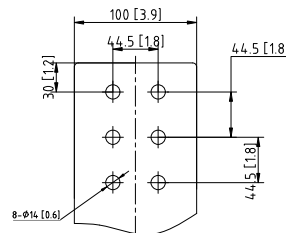
L.V. TERMINAL
