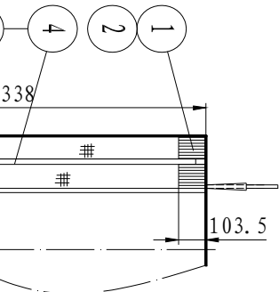
A(B, C)层间绝缘放置示意图
